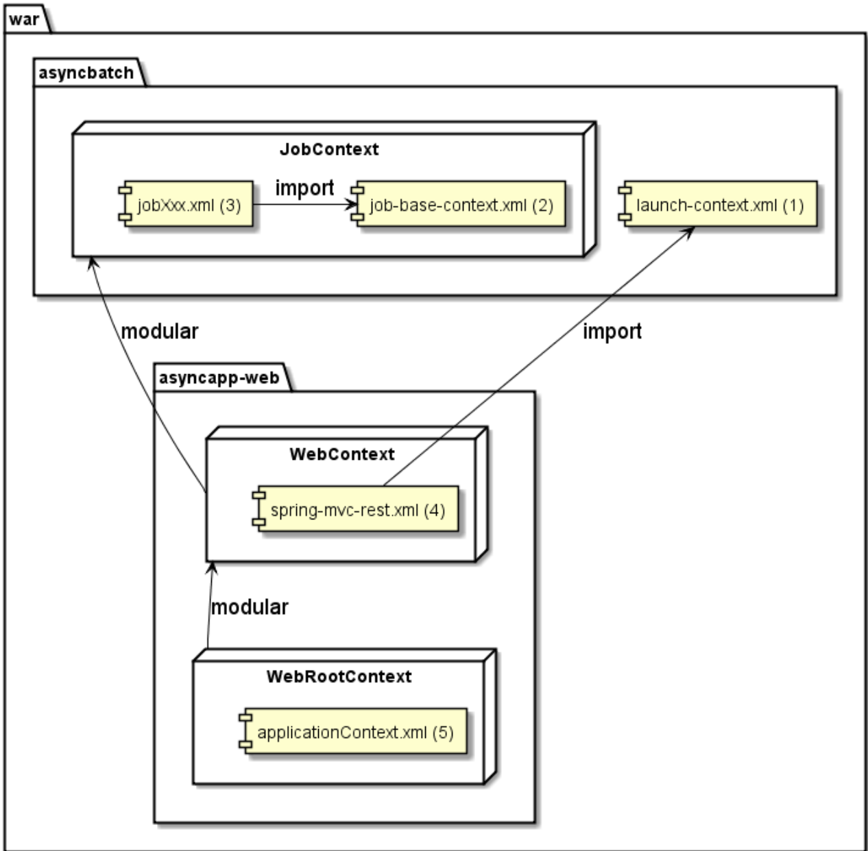
ApplicationContextの構成
