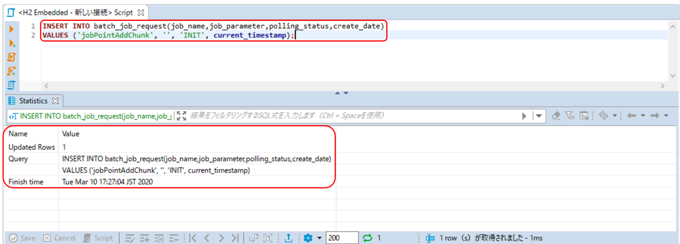
図 119. Execute SQL
