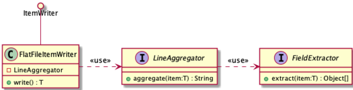
図 38. フラットファイルの出力を行うために使用するクラスの間連
