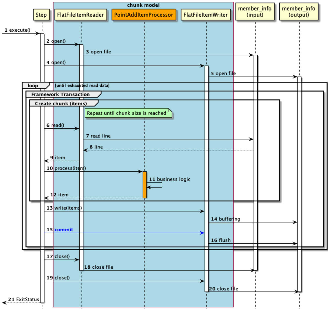
図 85. チャンクモデルのシーケンス図
