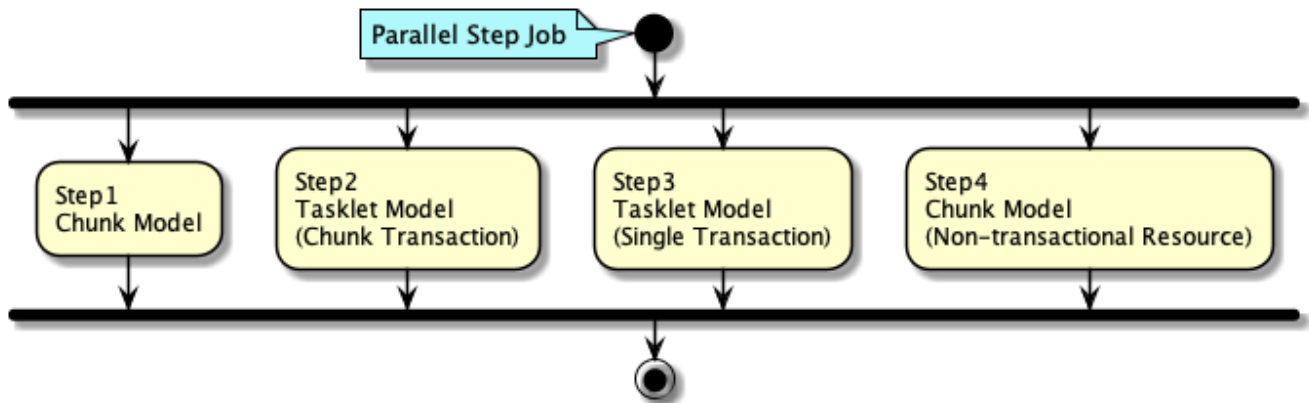
図 51. Parallel Stepの概要図
