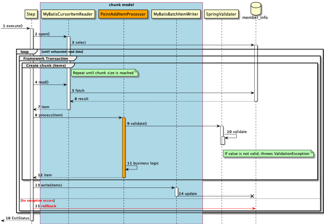
図 92. チャンクモデルのシーケンス図
