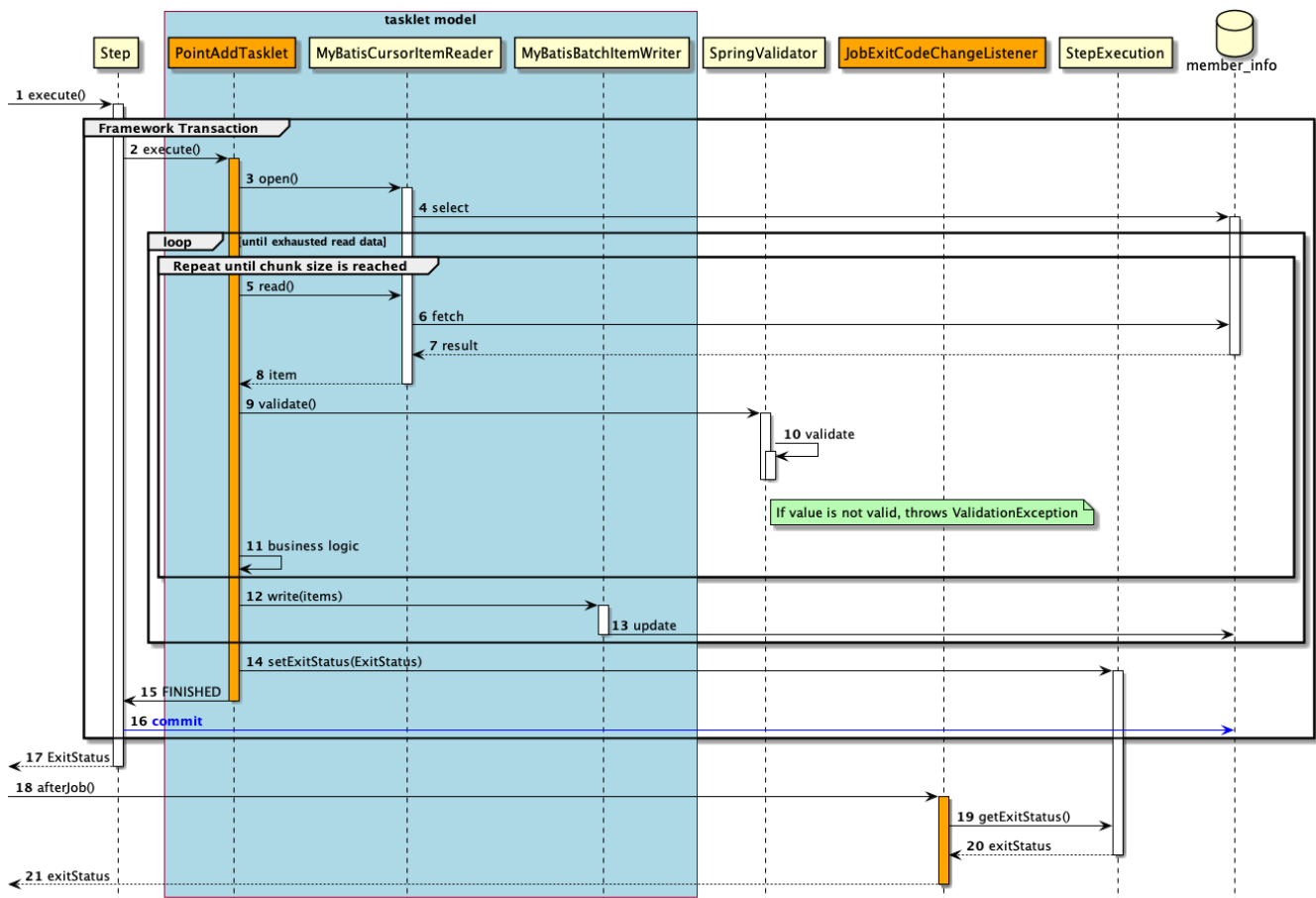
図 109. タスクレットモデルの処理シーケンス図
