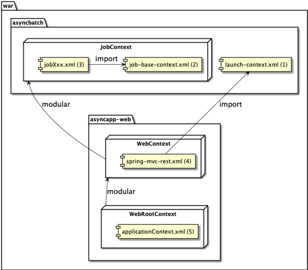
図 21. ApplicationContext の構成
