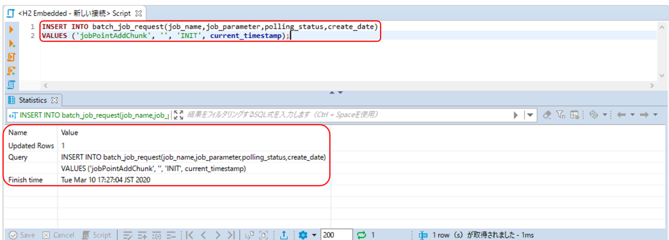
図 118. Execute SQL
