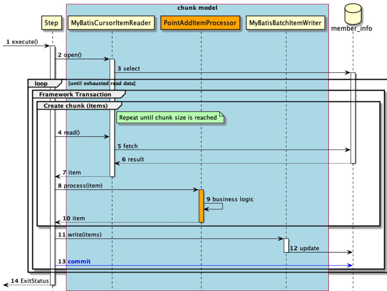
図 78. チャンクモデルのシーケンス図
