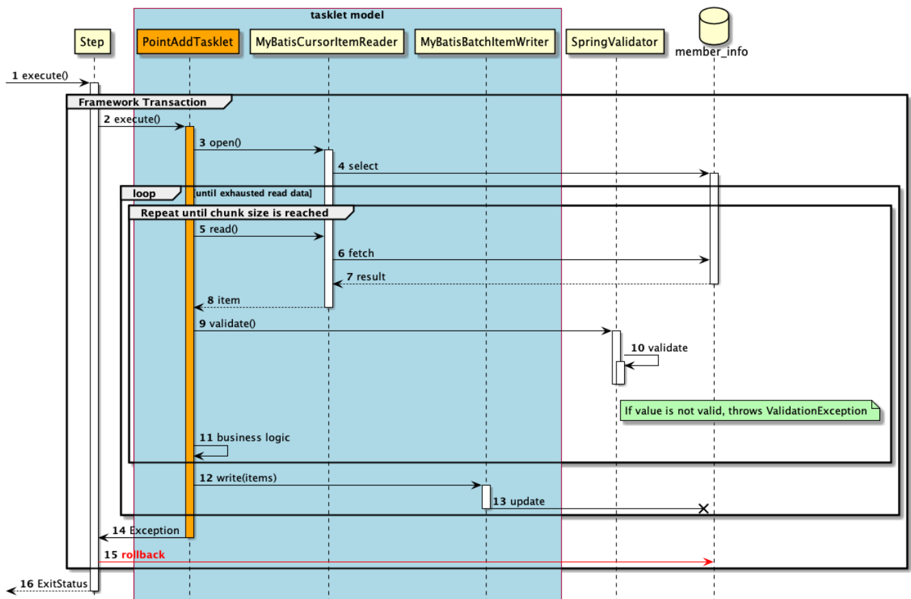
図 93. タスクレットモデルのシーケンス図
