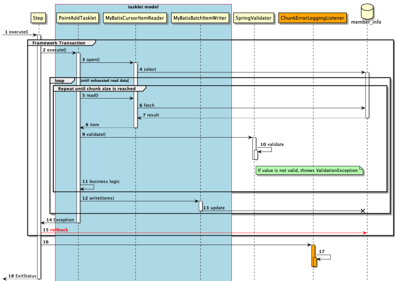
図 101. タスクレットモデルのシーケンス図
