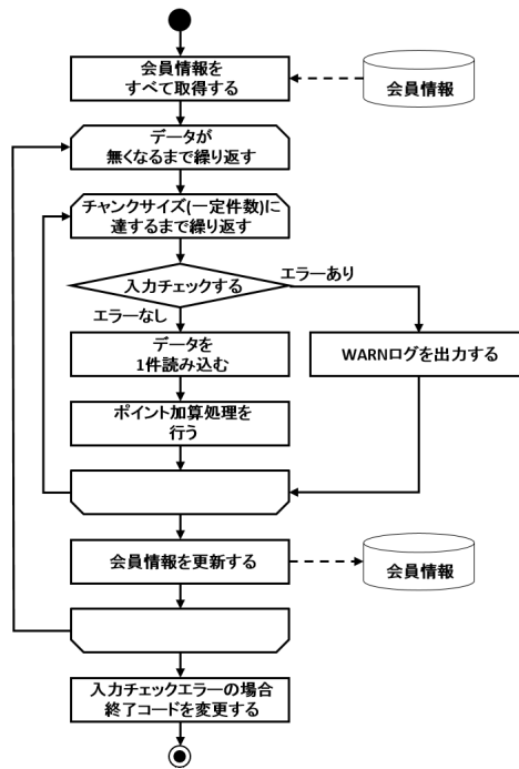
図 107. 例外ハンドリングを行うジョブの処理フロー
