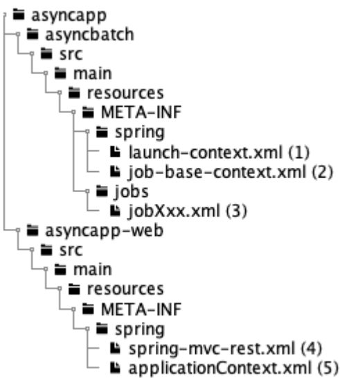
図 22. Bean定義ファイルの構成
