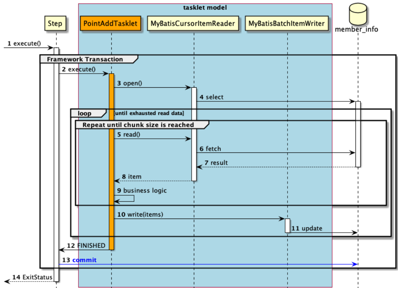
図 79. タスクレットモデルのシーケンス図
