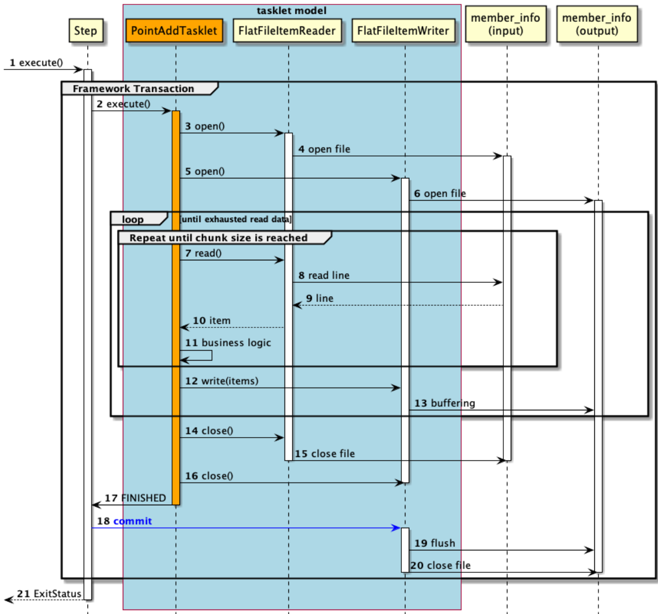
図 86. タスクレットモデルのシーケンス図
