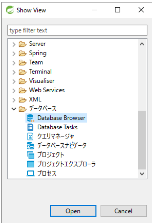
図 74. Show View
