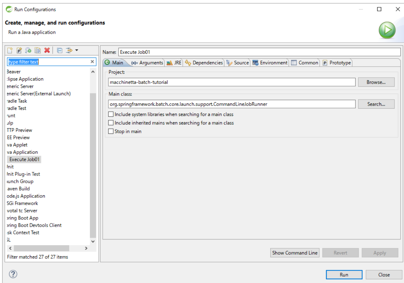
図 70. Run Job01
