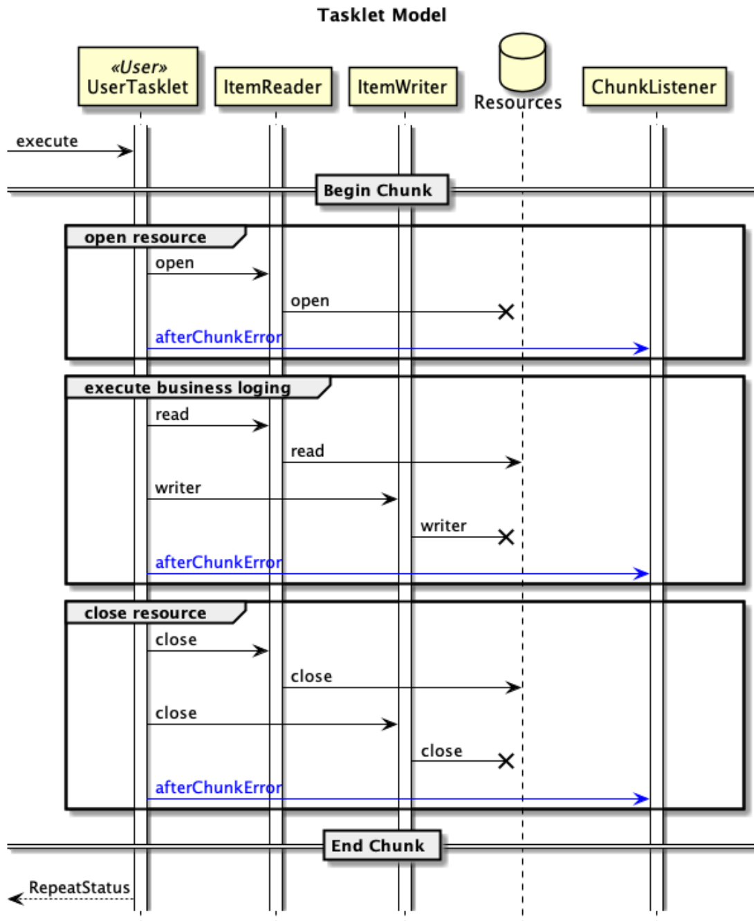
図 45. タスクレットモデルでの例外ハンドリング概略図
