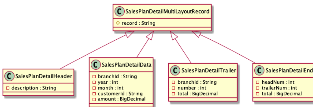
図 40. 変換対象クラスのクラス図
