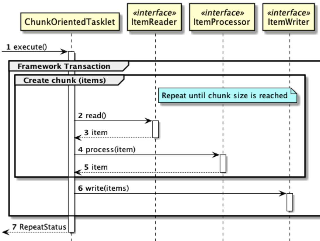
図 7. ChunkOrientedTasklet によるチャンク処理
