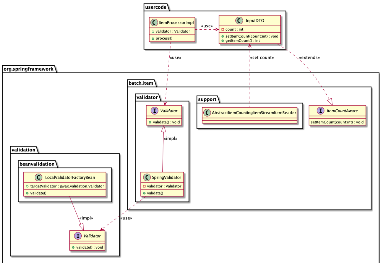
図 43. 入力チェックの関連クラス
