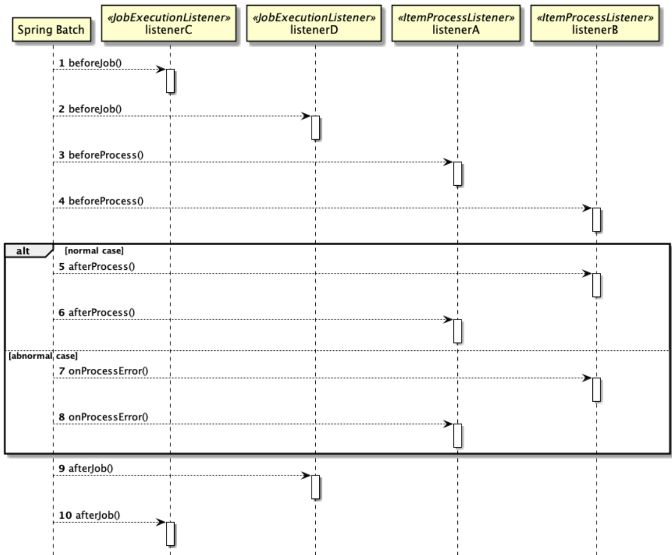
図 25. リスナーの起動順序
