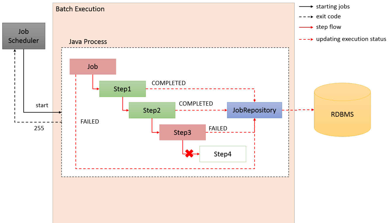
図 48. Macchinetta Batch 2.xによるフロー制御
