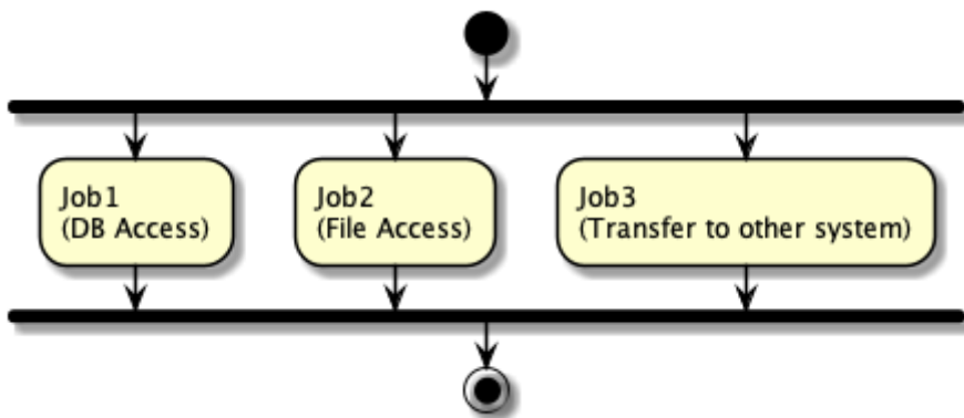
図 49. 並列処理の概略図
