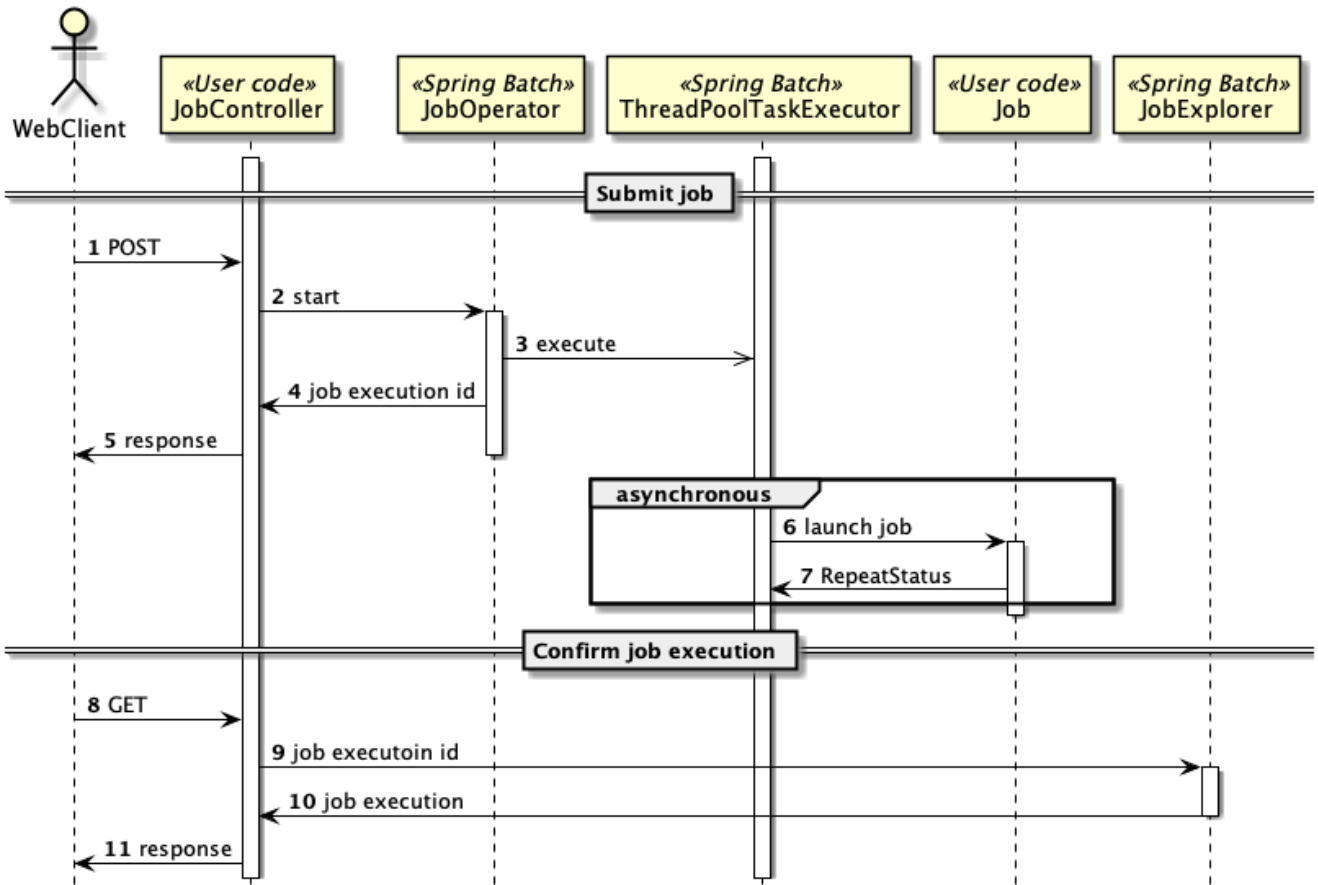
図 20. 非同期実行(Web コンテナ)のシーケンス図
