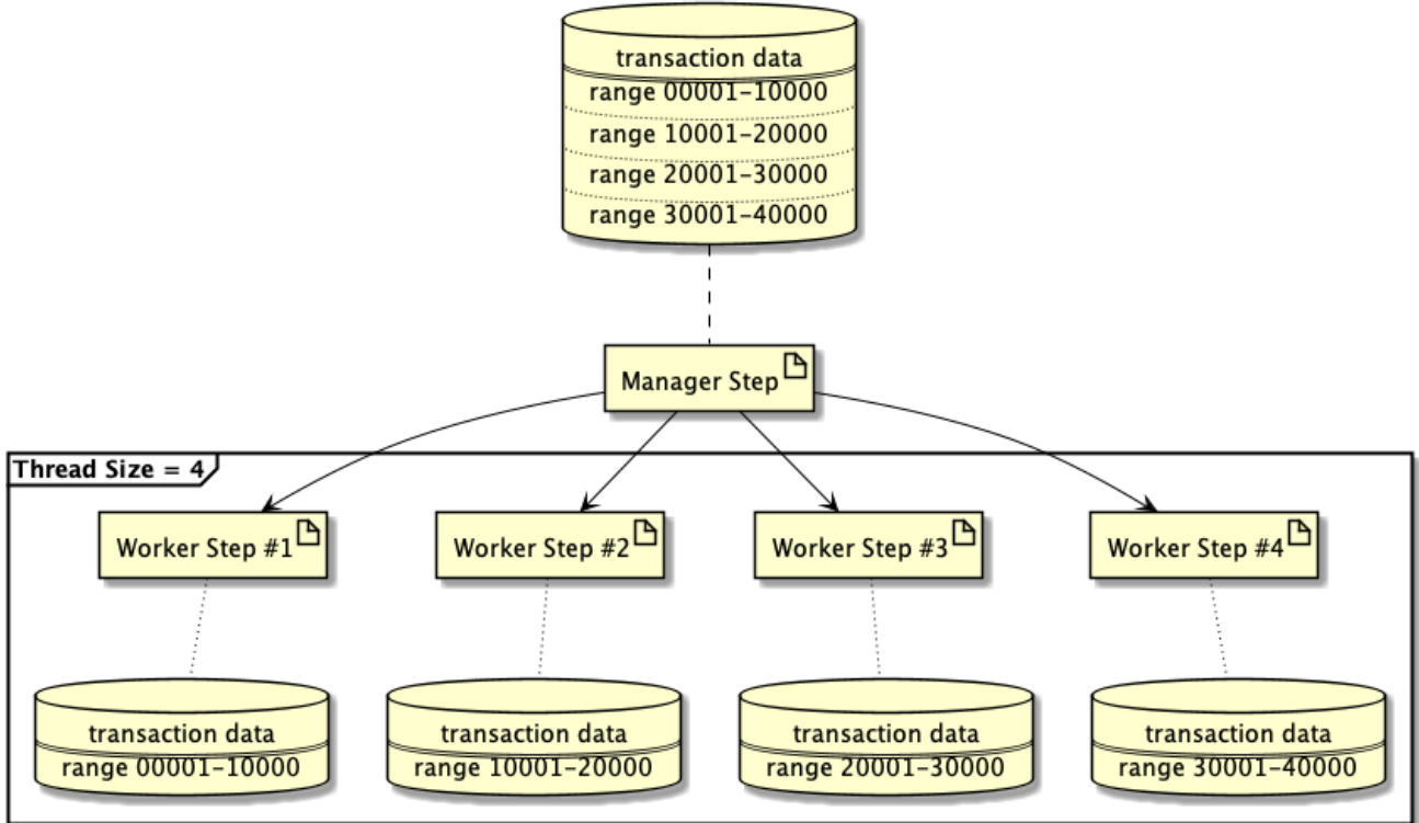
図 54. 処理イメージ図
