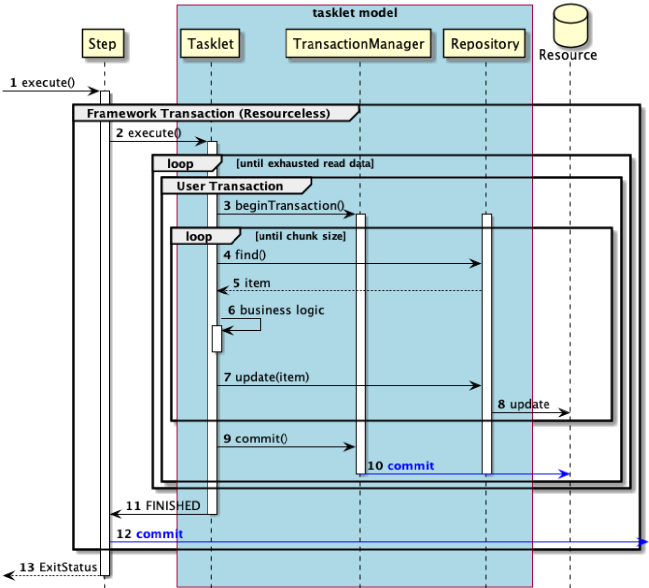
図 30. 正常系のシーケンス図
