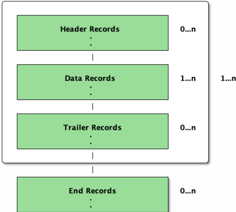
図 35. マルチフォーマットのレコード構成図
