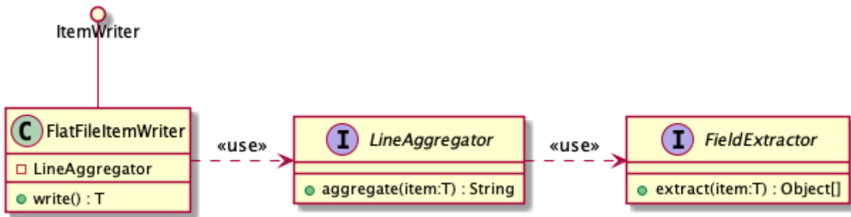
図 38. フラットファイルの出力を行うために使用するクラスの関連
