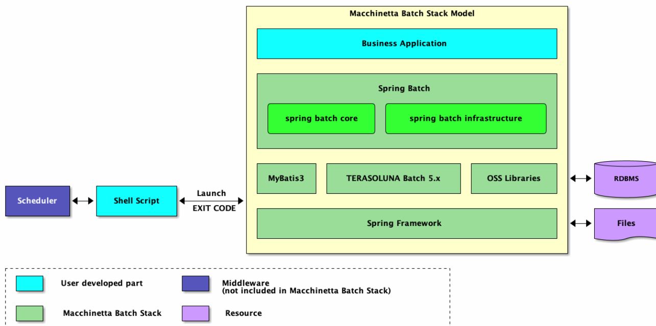
図 9. Macchinetta Batch Framework (2.x)の構成概略図
