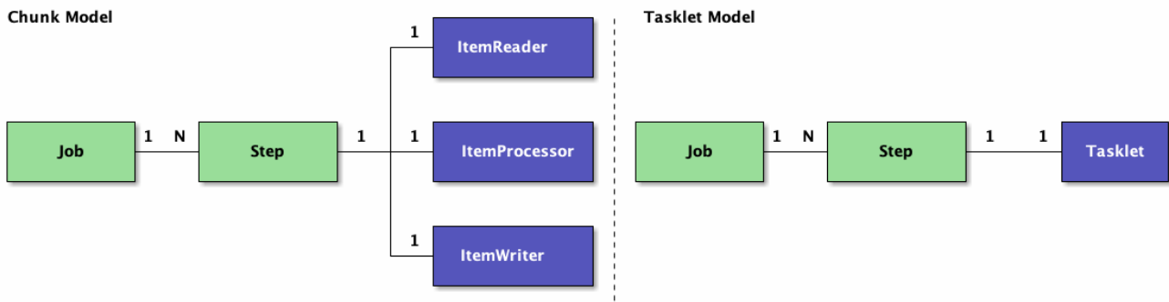
図 10. ジョブの構成概略図
