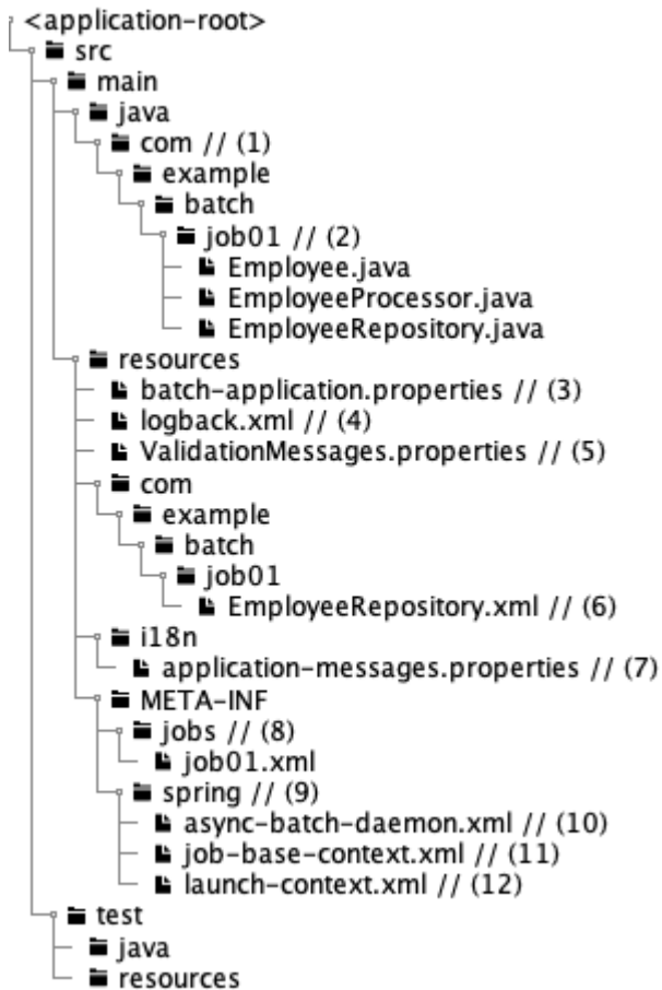
図 14. プロジェクトのディレクトリ構造
