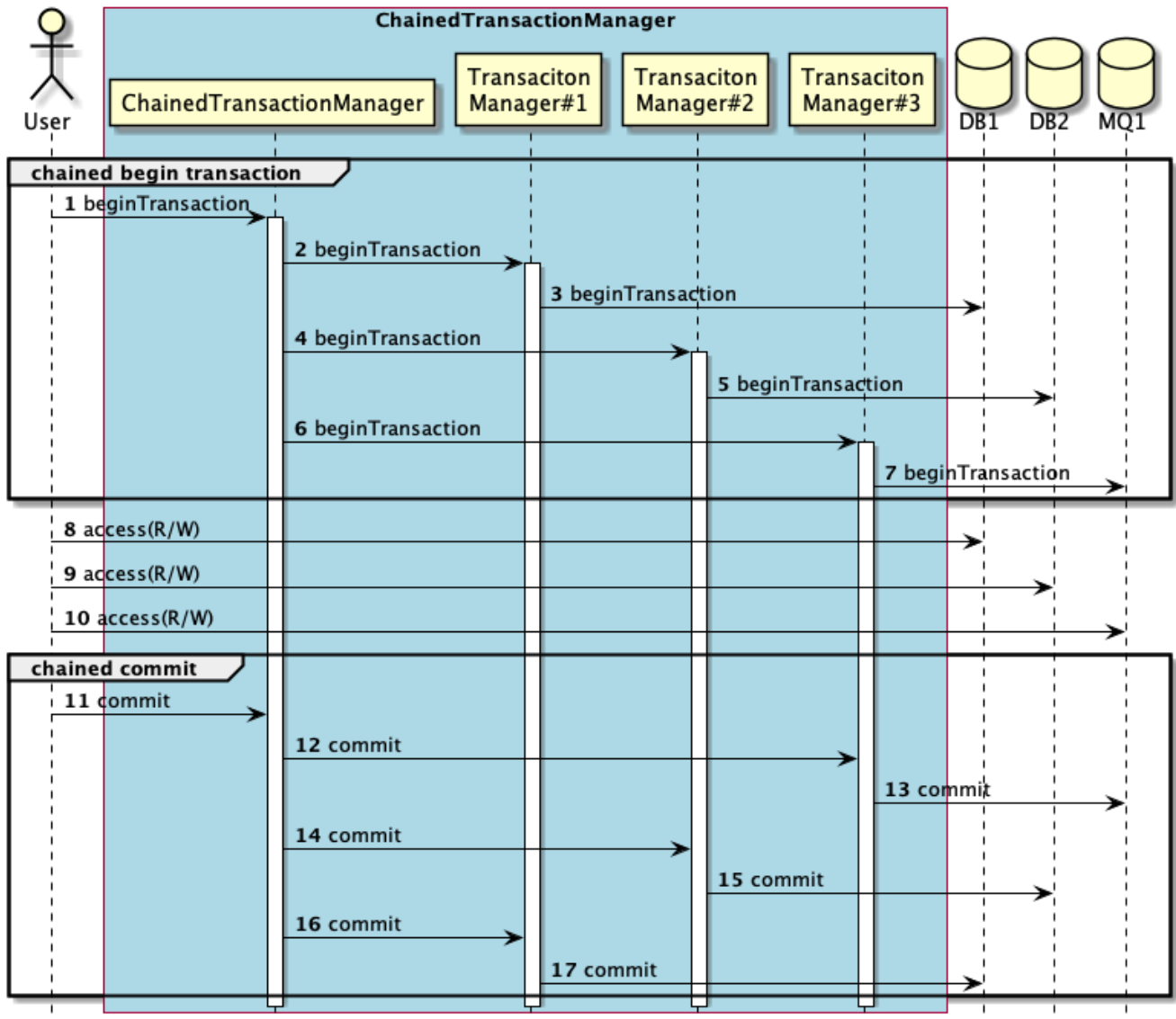
図 34. Best Efforts 1PCパターンの概念図
