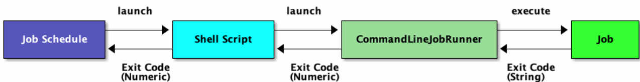
図 11. 同期実行概略図
