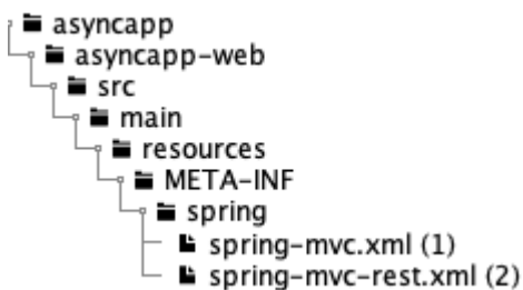
図 24. 空白プロジェクトから追加・削除するBean定義ファイル
