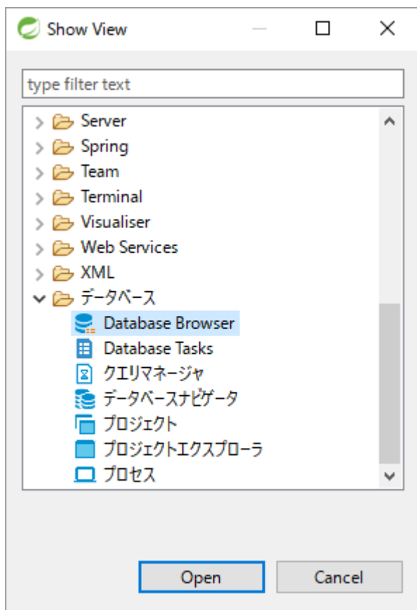
図 75. Show View
