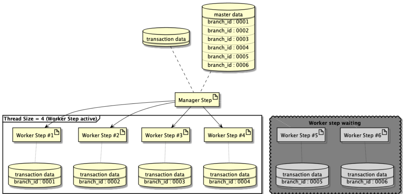
図 53. 処理イメージ図
