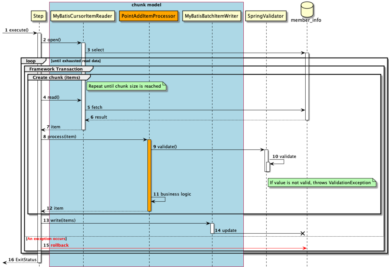
図 93. チャンクモデルのシーケンス図
