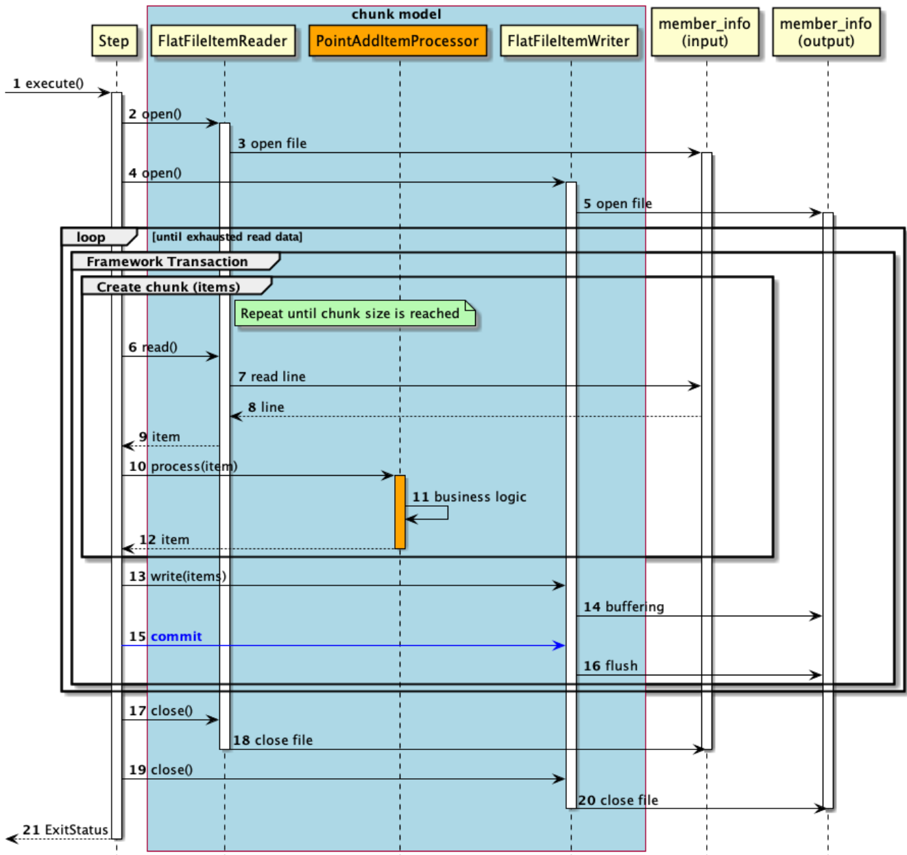
図 86. チャンクモデルのシーケンス図
