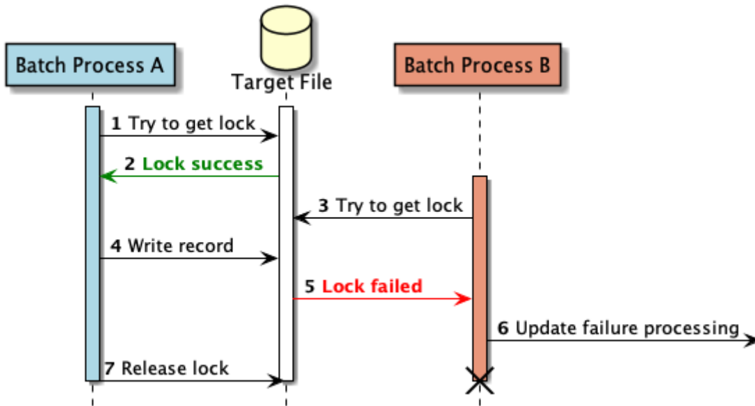
図 41. ファイルロックの実施イメージ
