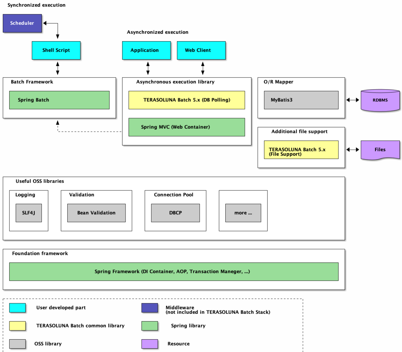
図 2. Software Framework構成要素の概略図
