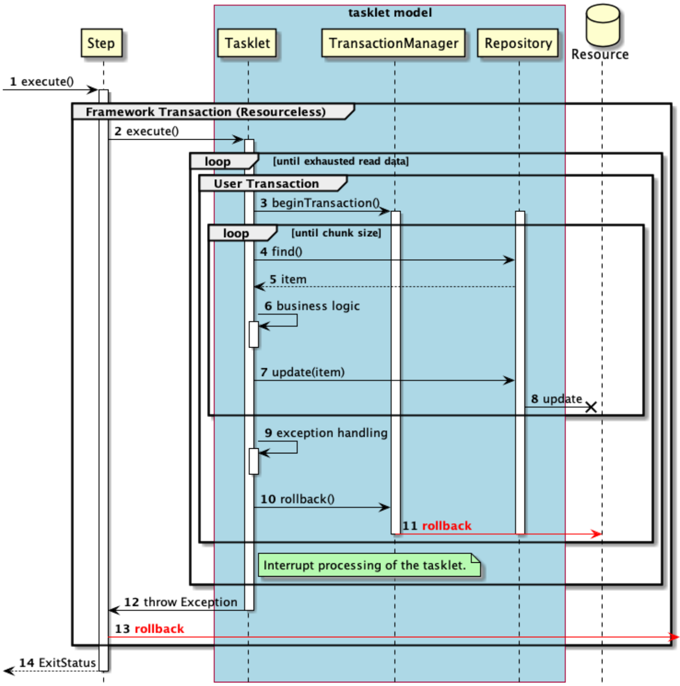
図 31. 異常系のシーケンス図
