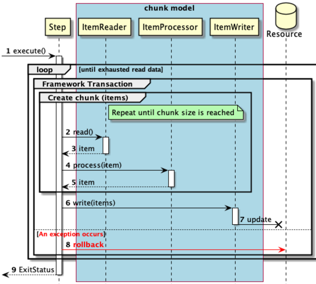
図 27. 異常系のシーケンス図
