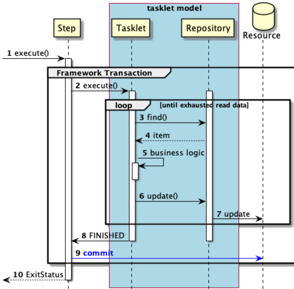
図 28. 正常系のシーケンス図
