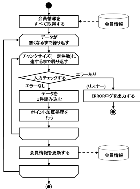
図 100. 例外ハンドリングを行うジョブの処理フロー
