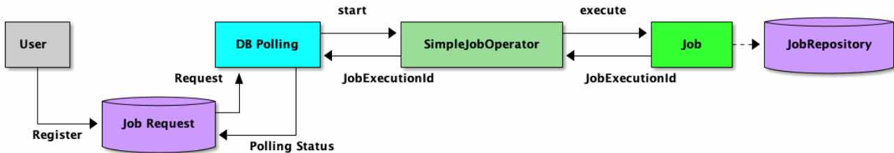
図 12. DBポーリング概略図
