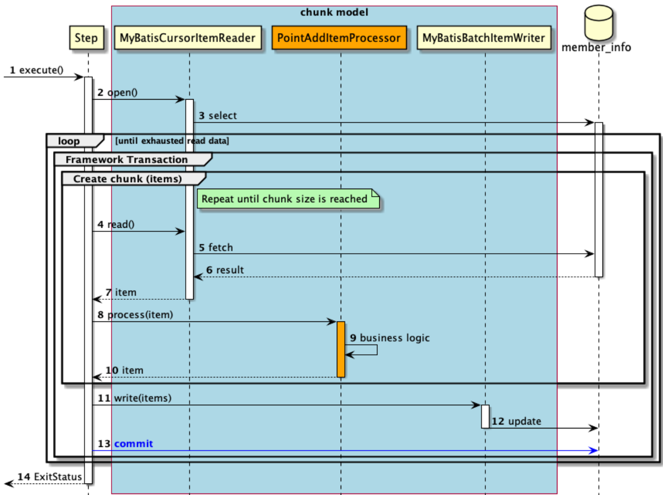
図 79. チャンクモデルのシーケンス図
