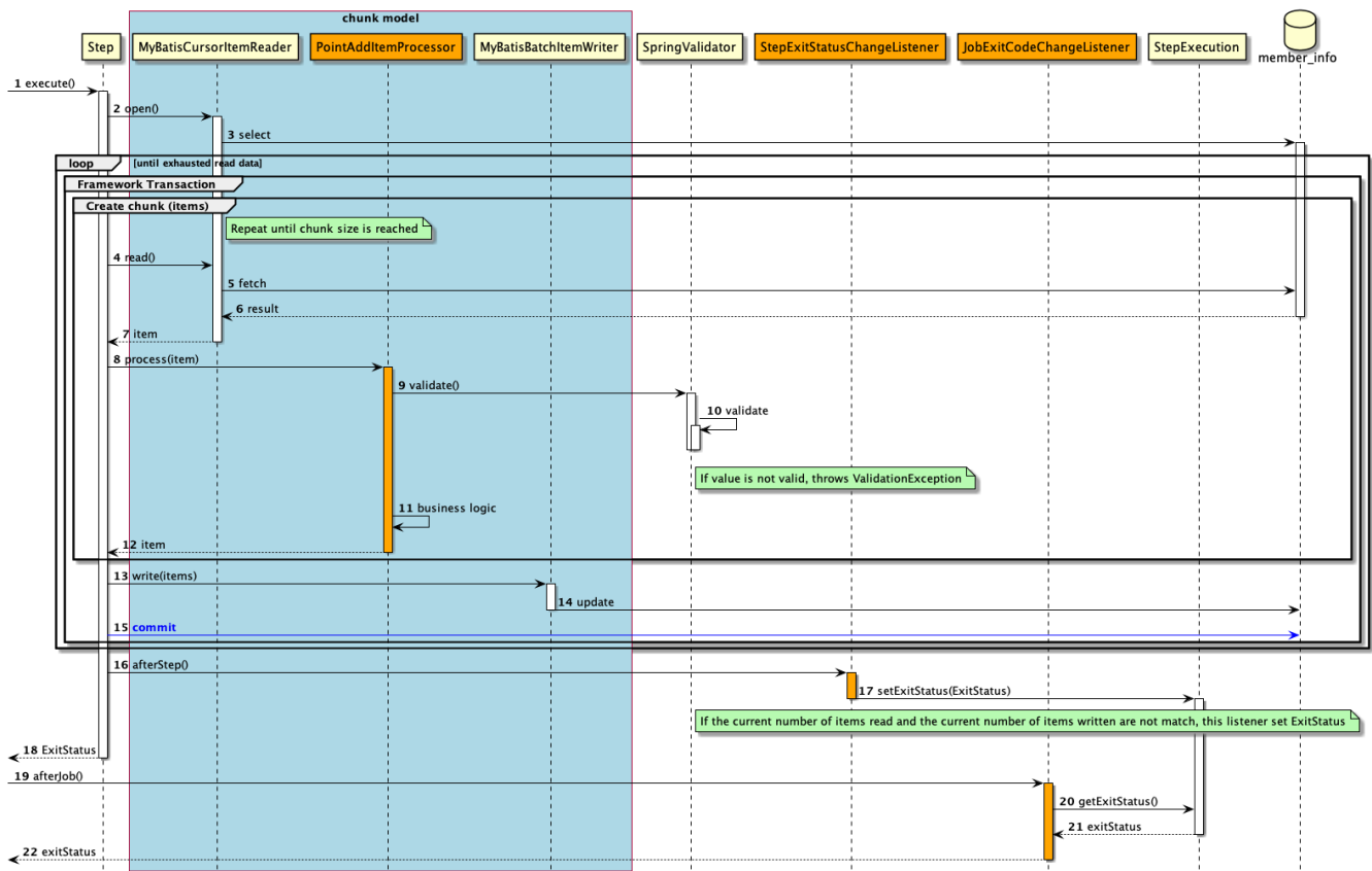
図 109. チャンクモデルのシーケンス図
