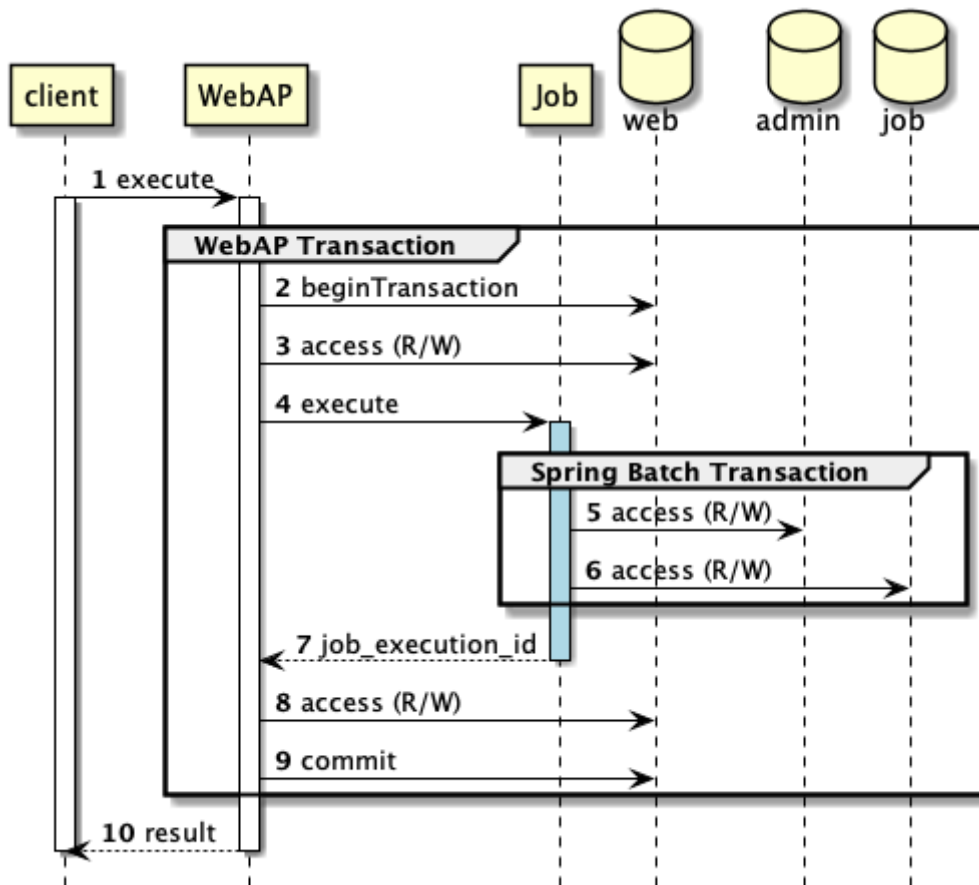
図 33. WebAPサーバ処理のトランザクション
