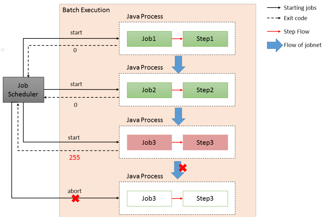
図 47. ジョブスケジューラによるフロー制御
