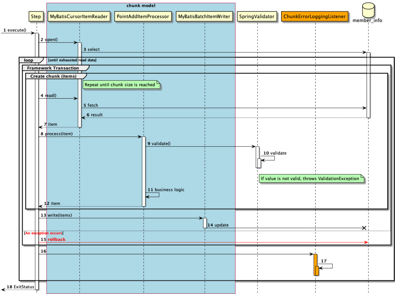
図 101. チャンクモデルのシーケンス図
