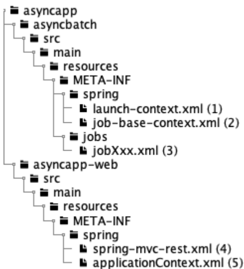
図 22. Bean定義ファイルの構成
