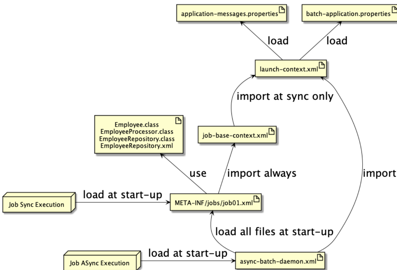
図 15. 各ファイルの関連図
