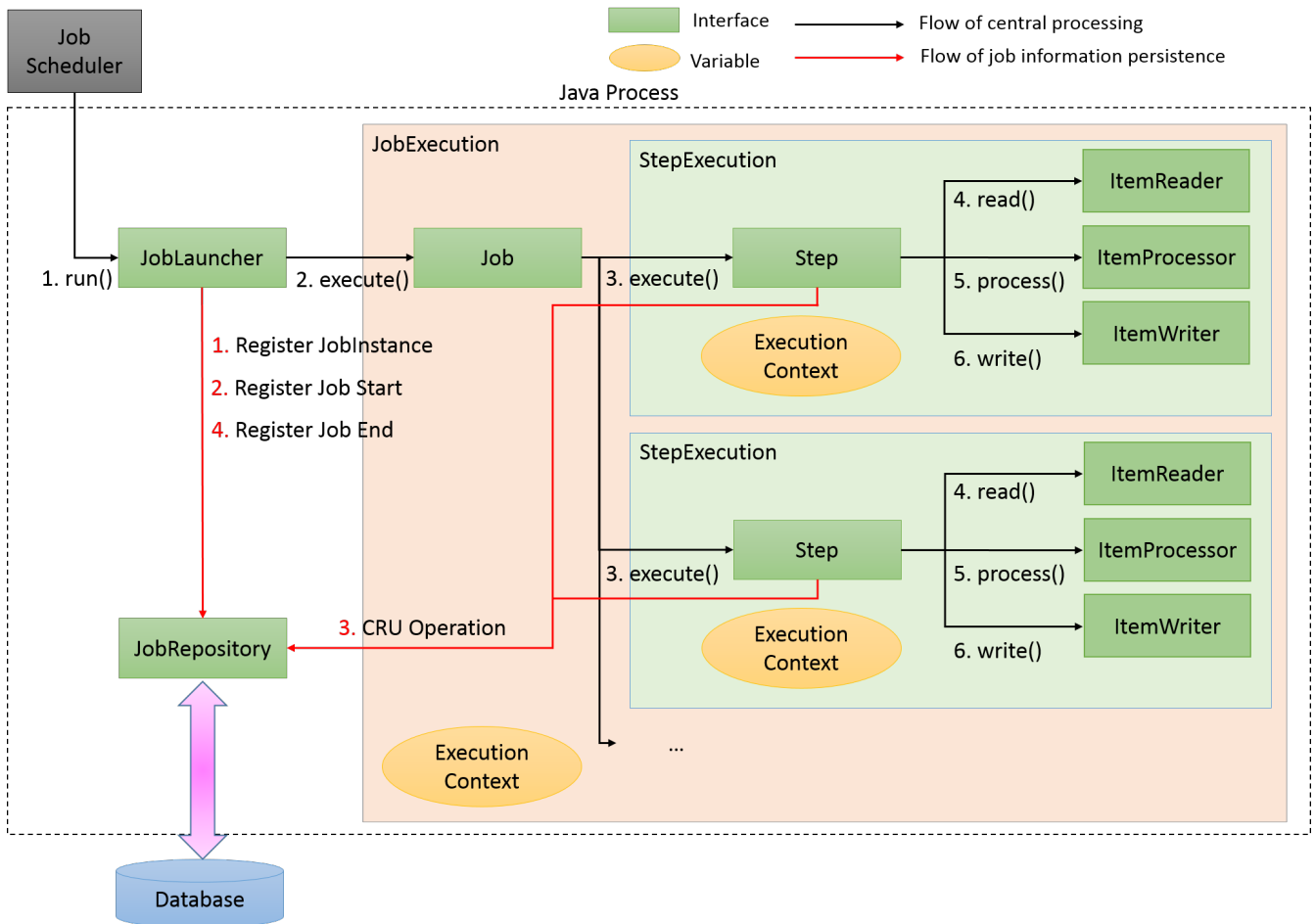
図 4. Spring Batchの主な構成要素と処理全体の流れ
