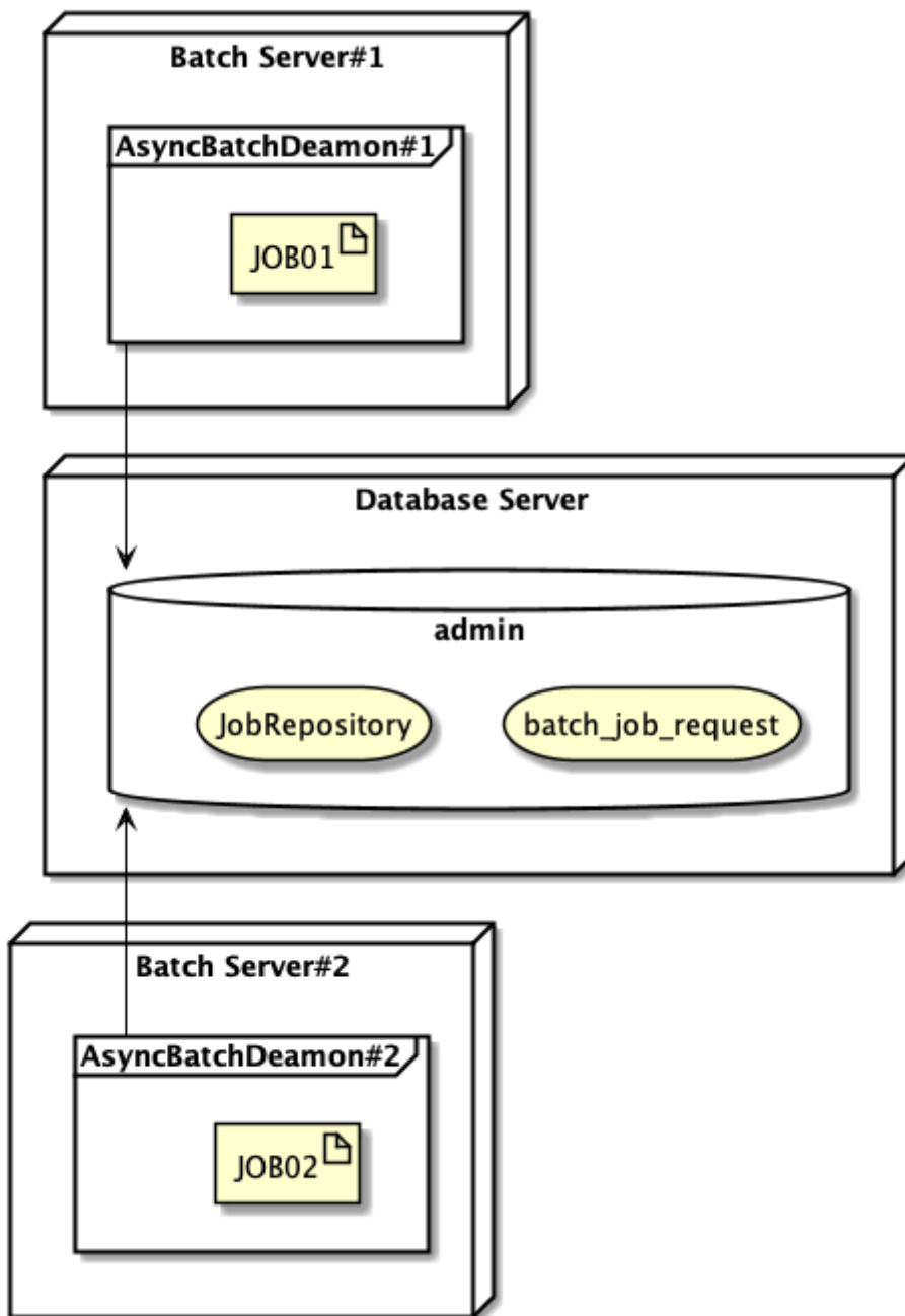
図 19. 複数起動の概略図
