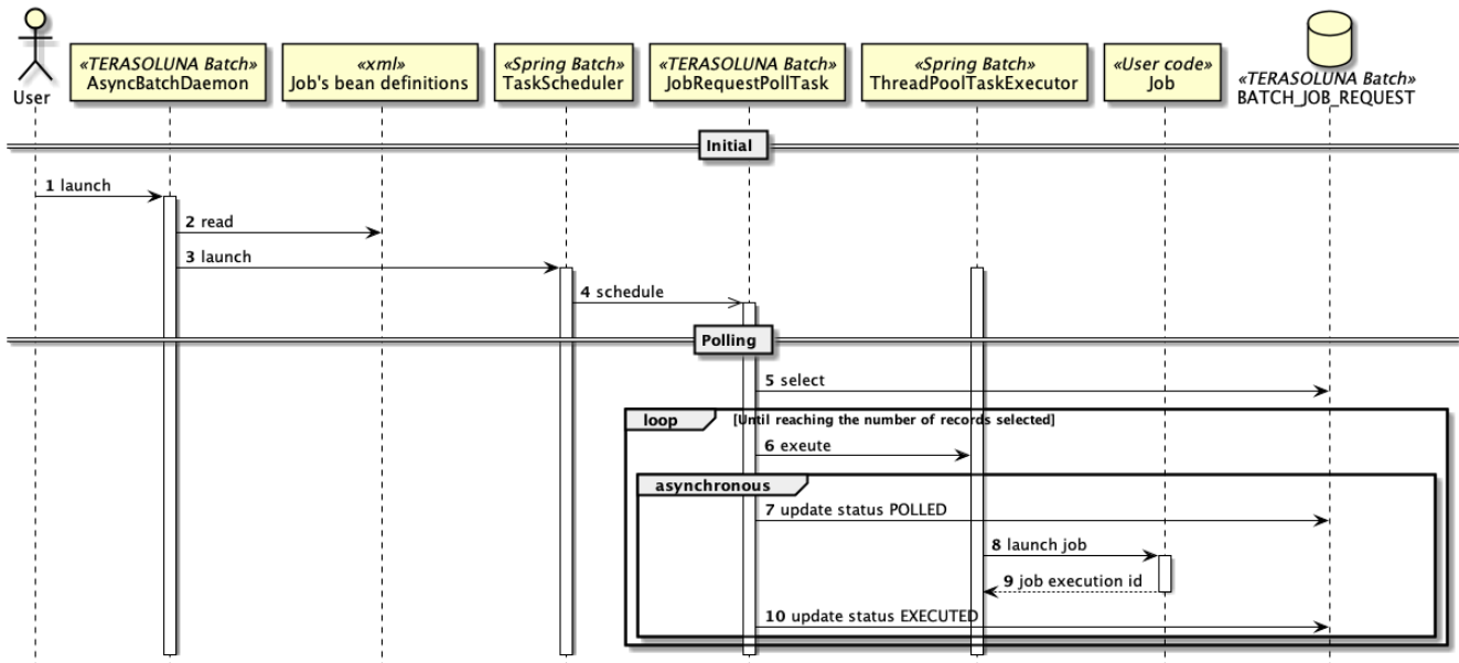
図 18. DBポーリングのシーケンス図
