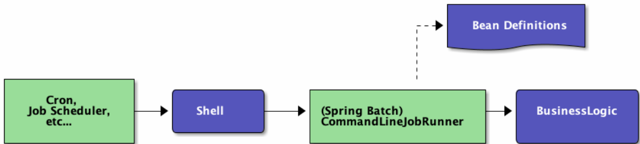
図 16. 同期実行の概要
