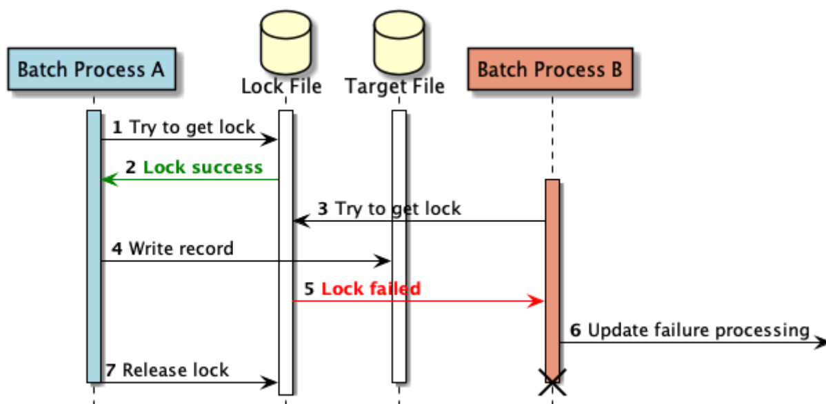
図 42. ロック用ファイルを用いたファイルロックの実施イメージ
