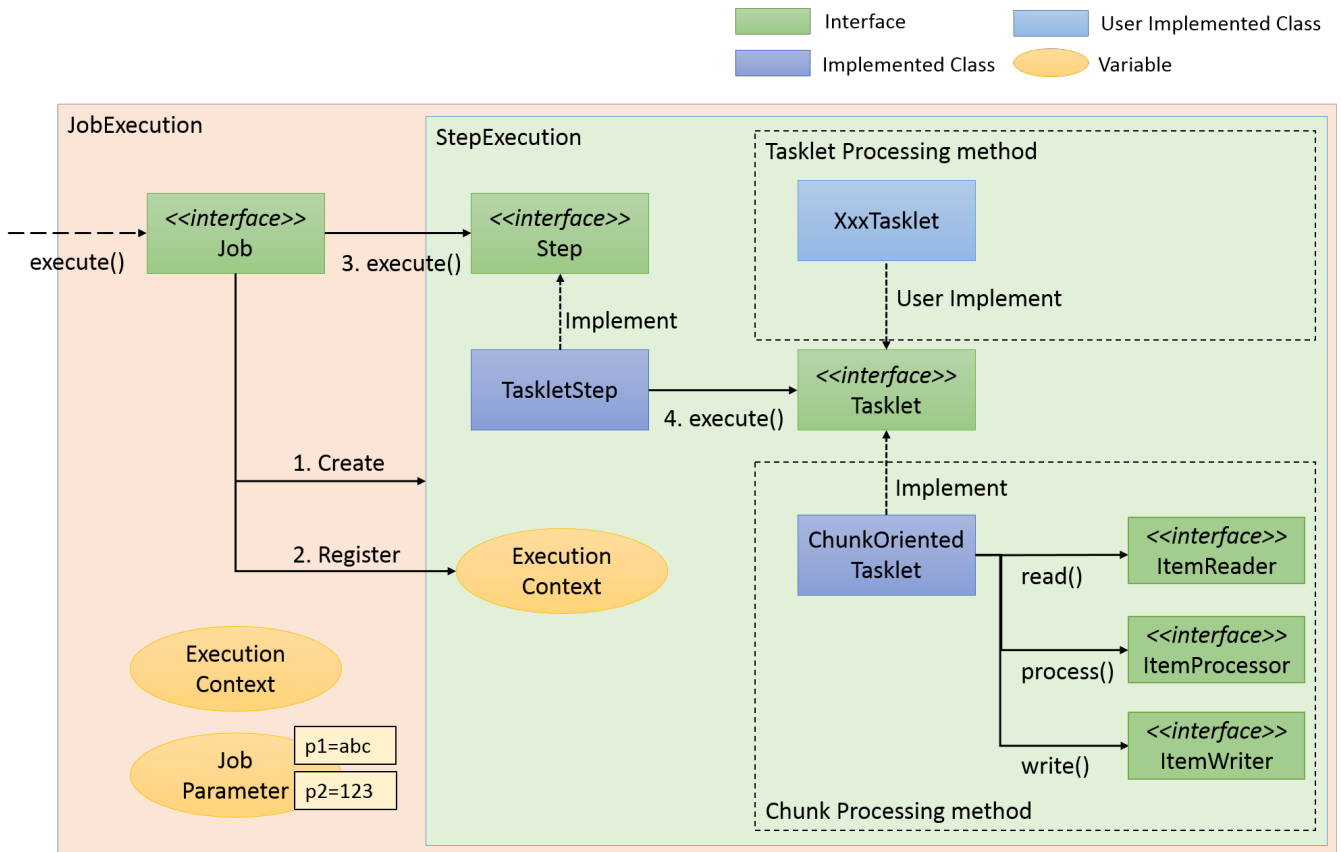
図 6. StepからTaskletへの流れ
