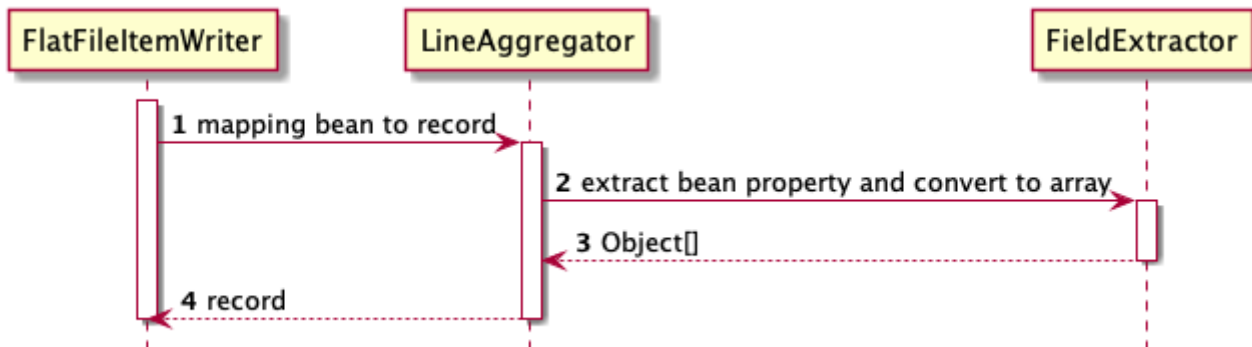
図 39. 各コンポーネントの呼び出し関係
