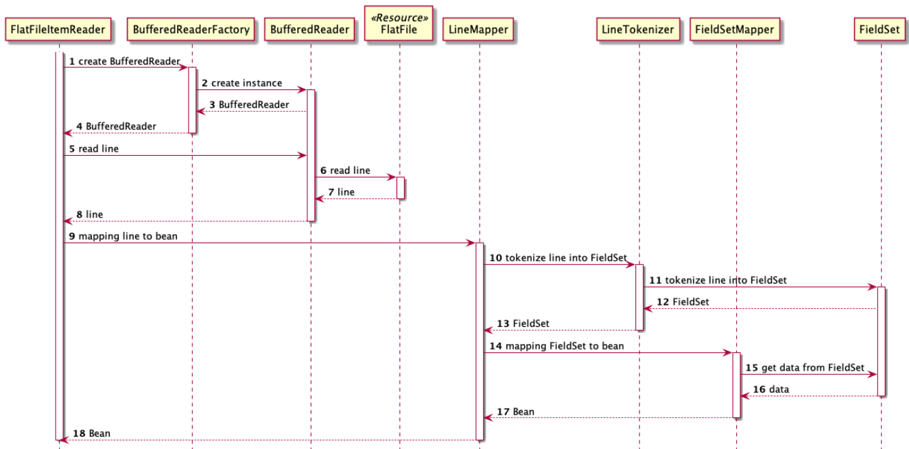
図 37. 各コンポーネントの呼び出し関係
