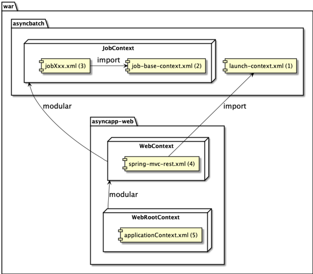
図 21. ApplicationContext の構成
