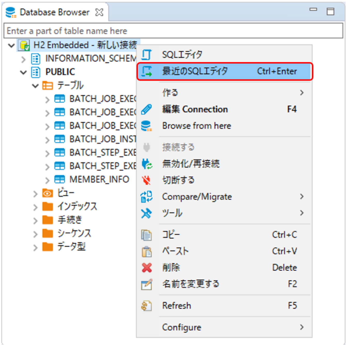
図 118. SQL Editor
