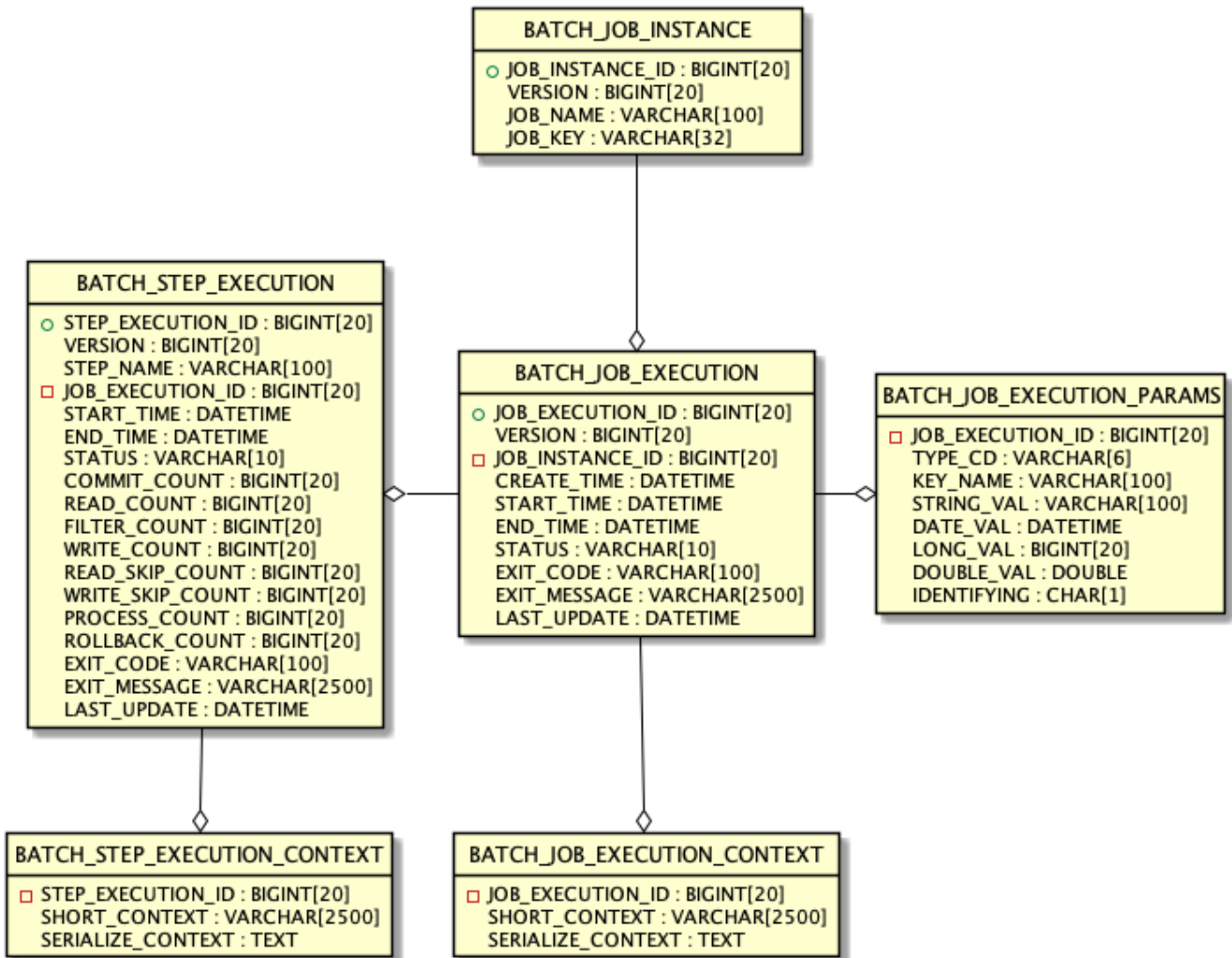
図 8. ER図
