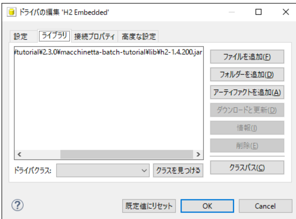
図 65. Edit Library
