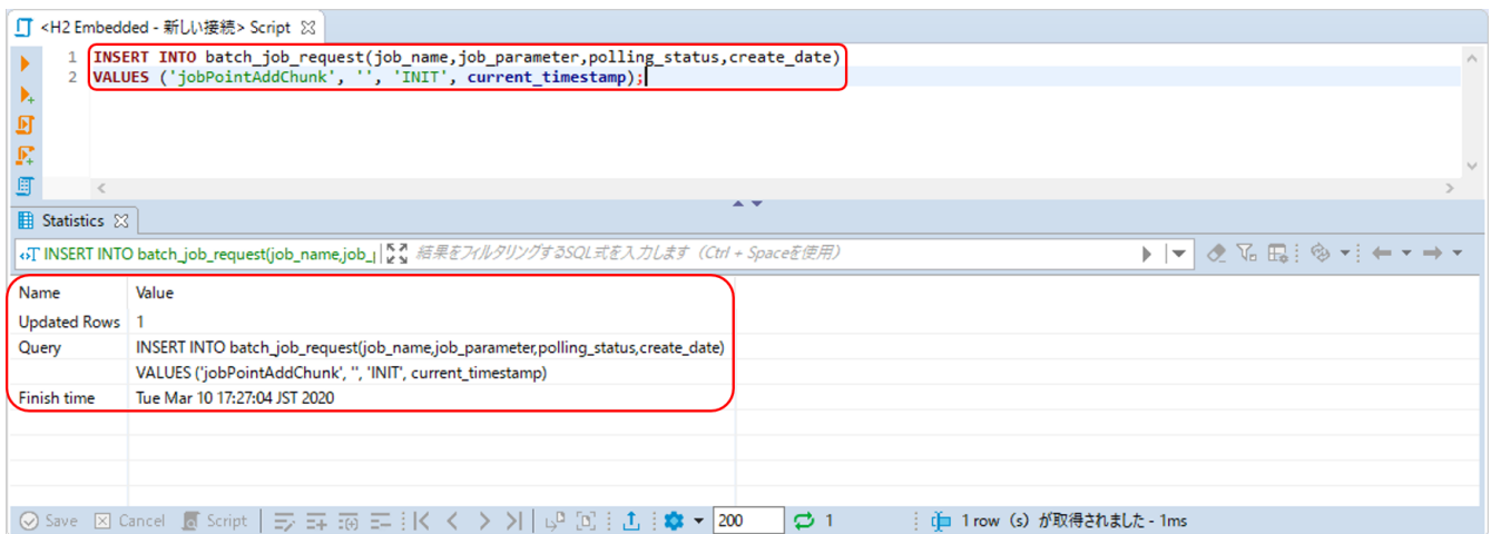
図 119. Execute SQL
