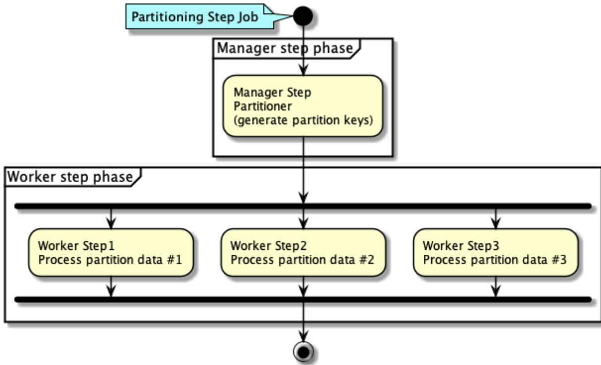
図 52. Partitioning Stepの概要図
