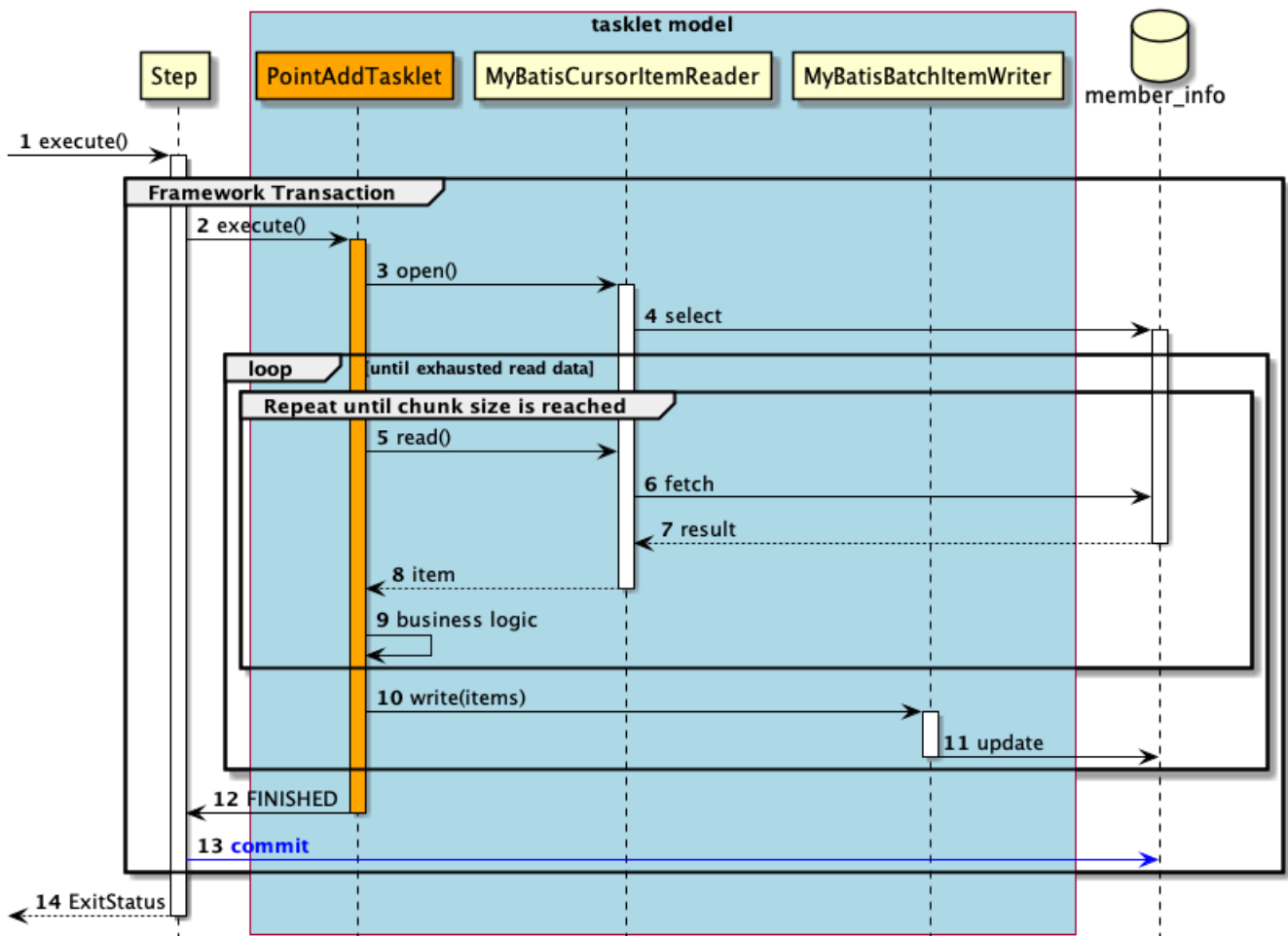
図 80. タスクレットモデルのシーケンス図
