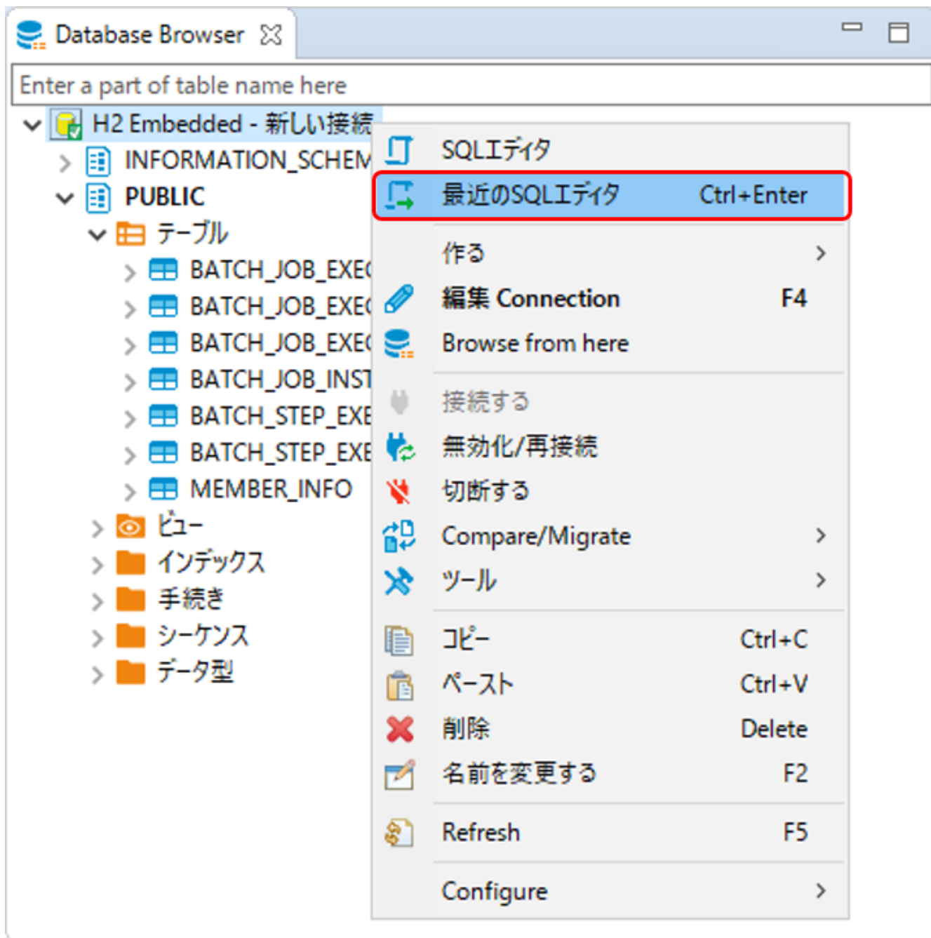
図 118. SQL Editor
