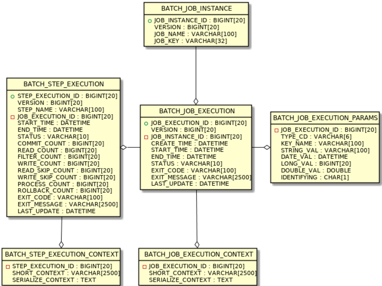
図 8. ER図
