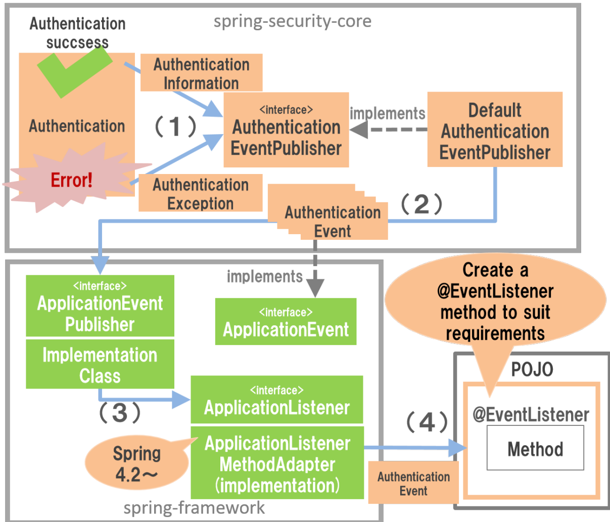
図5 イベント通知の仕組み
