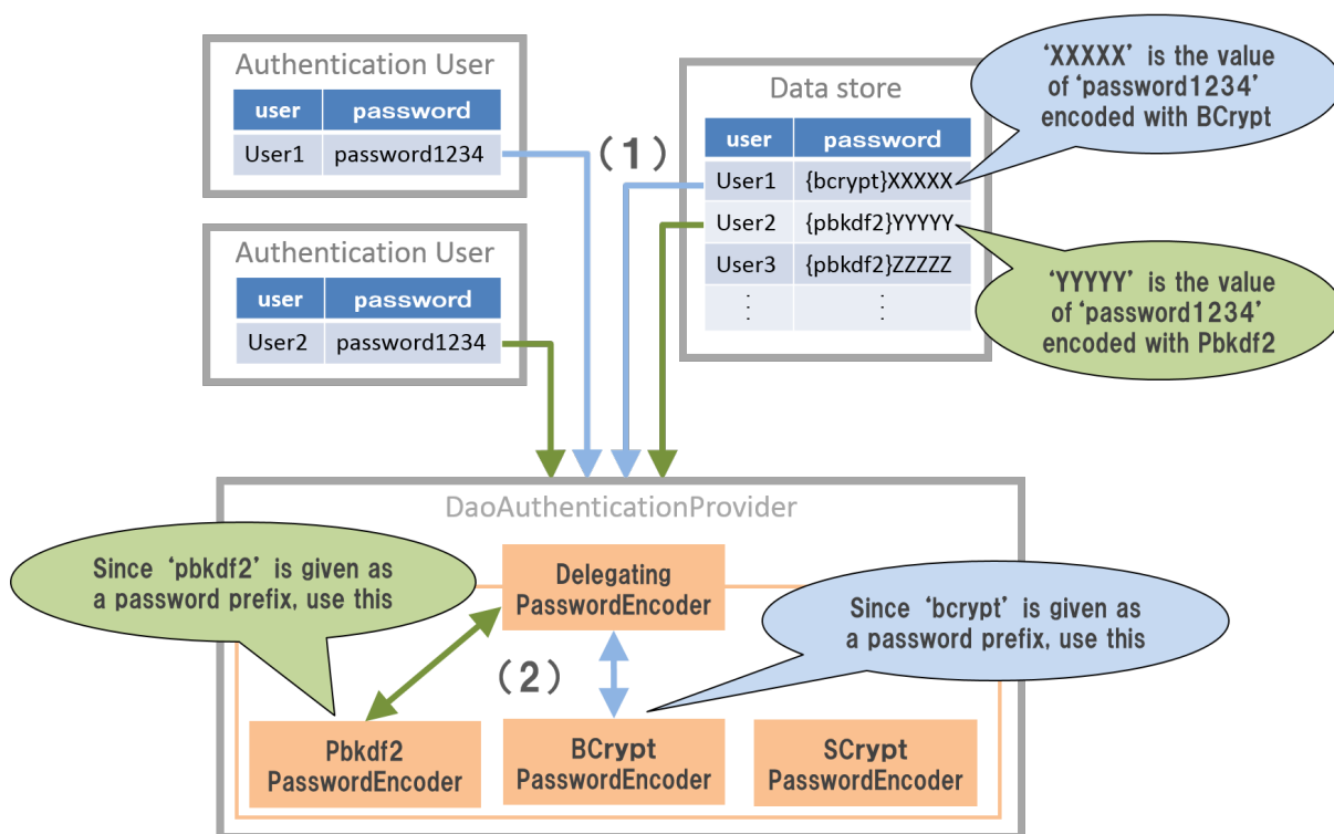
図 5 DelegatesPasswordEncoder の解説
