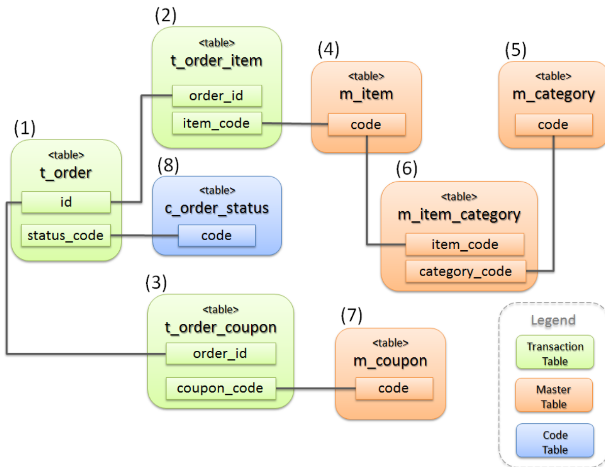
図 6 Picture - ER diagram
