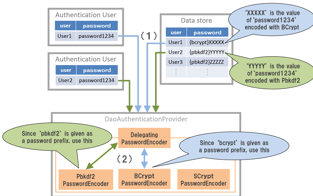
図 5 DelegatingPasswordEncoder の解説
