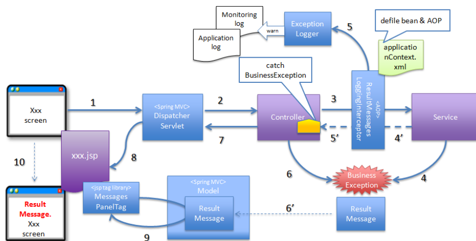
図 4.9 図-リクエスト単位で Controller クラスがハンドリングする場合の基本フロー
