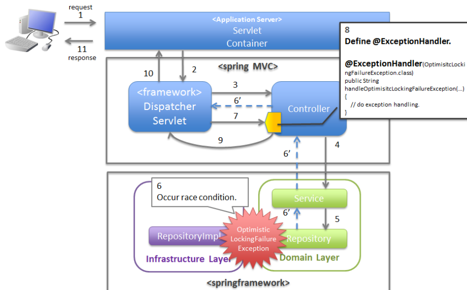
図 4.4 図-ユースケースのやり直し (先頭からのやり直し) を促す場合のハンドリング方法
