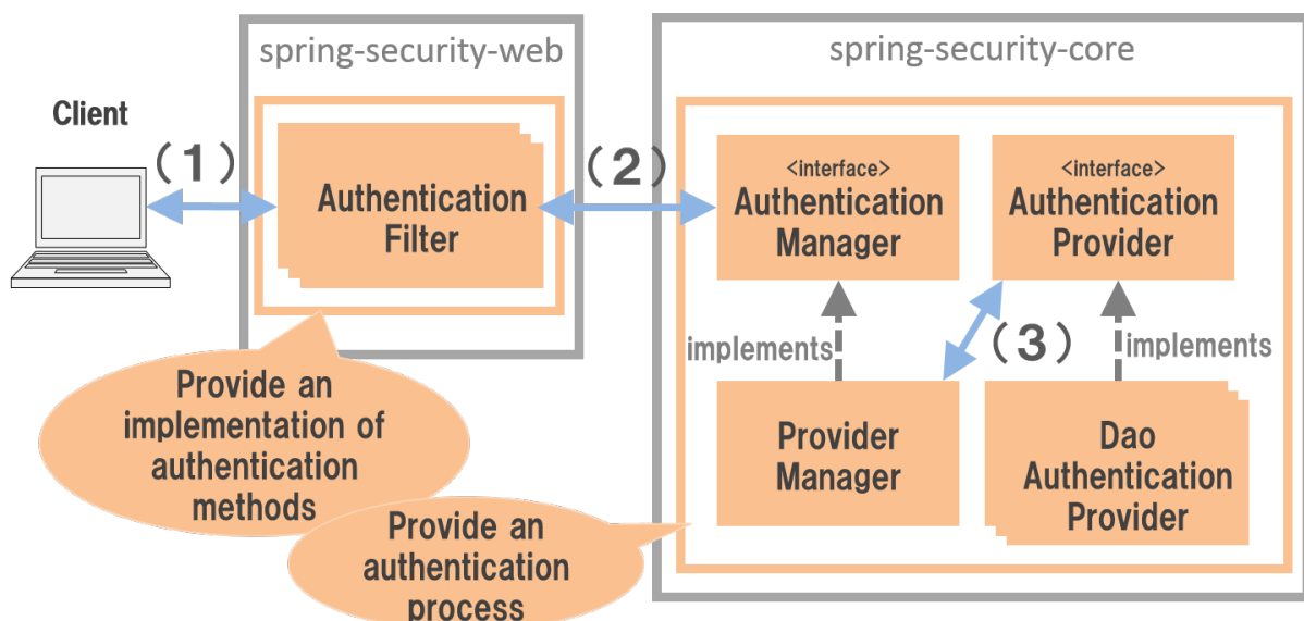
図 9.2 認証処理のアーキテクチャ
