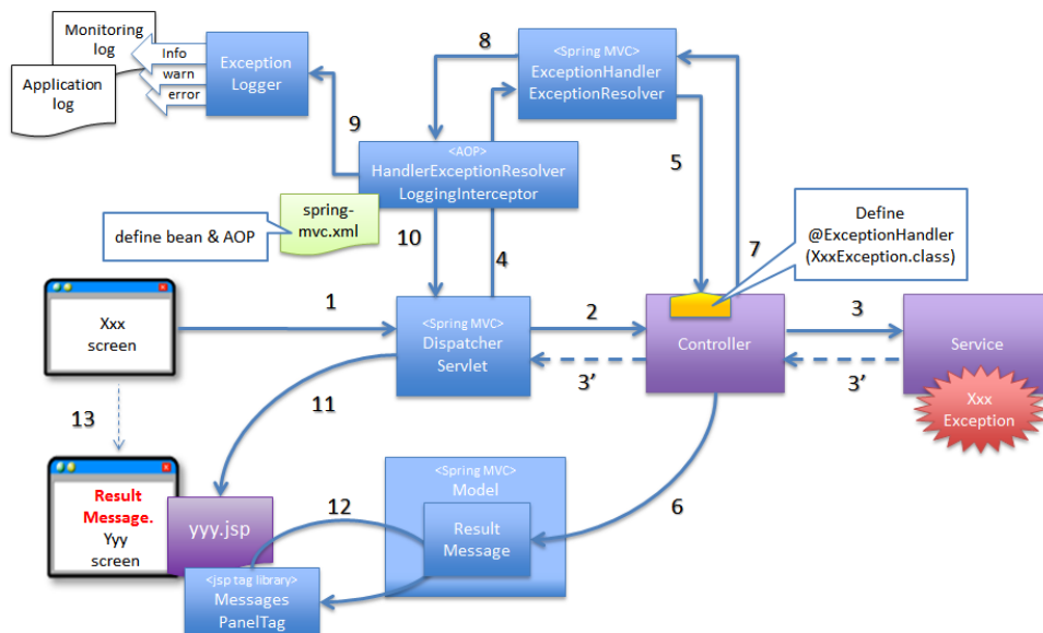
図 4.10 図-ユースケース単位で、Controller クラスがハンドリングする場合の基本フロー
