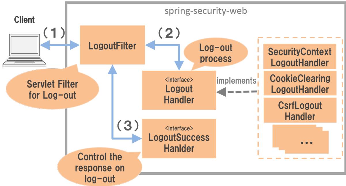
図 9.6 ログアウト処理の仕組み
