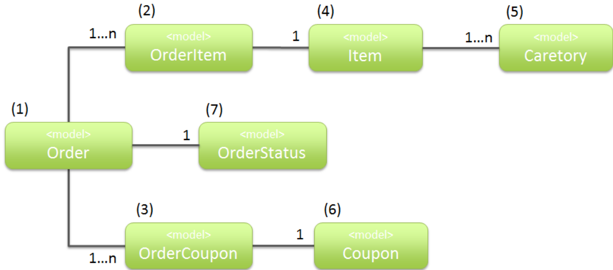
図 6.7 Picture - Class(JavaBean) diagram
