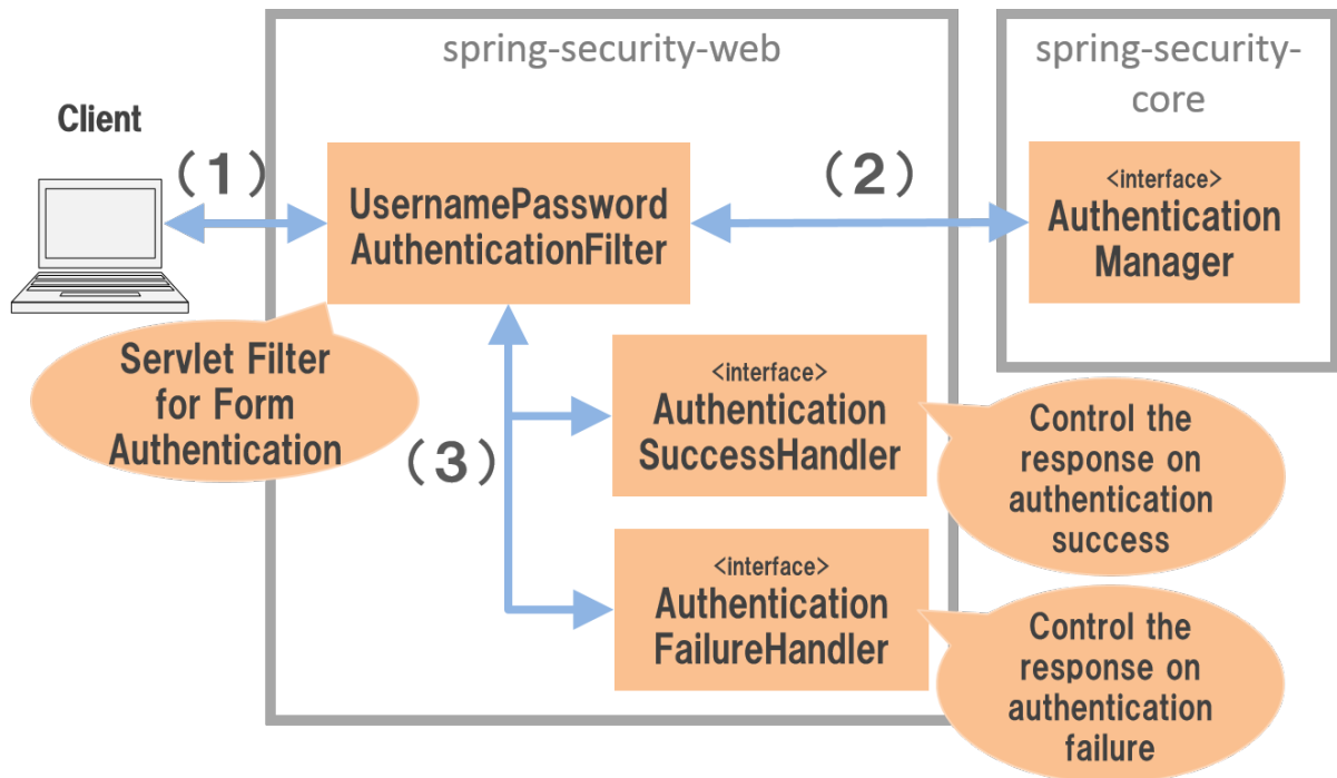
図 9.3 フォーム認証の仕組み
