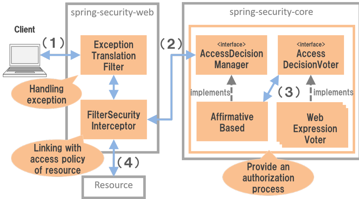
図 9.7 認可処理のアーキテクチャ
