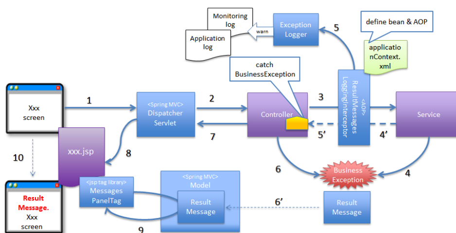
図 4.9 図-リクエスト単位で Controller クラスがハンドリングする場合の基本フロー
