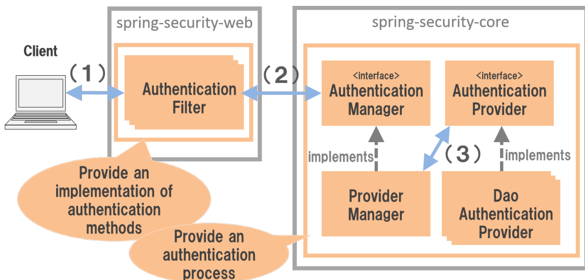
図 9.2 認証処理のアーキテクチャ
