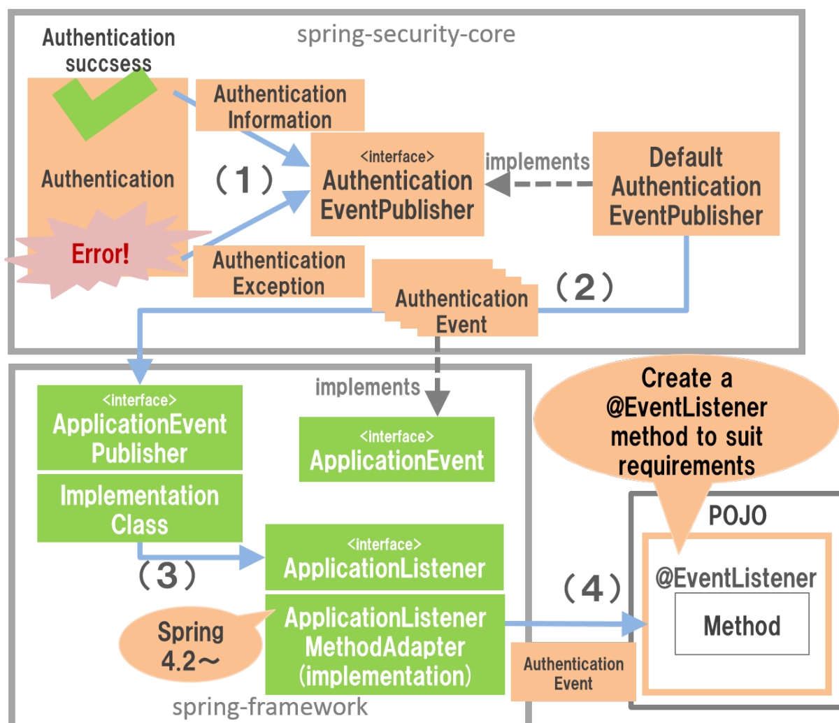
図 9.5 イベント通知の仕組み
