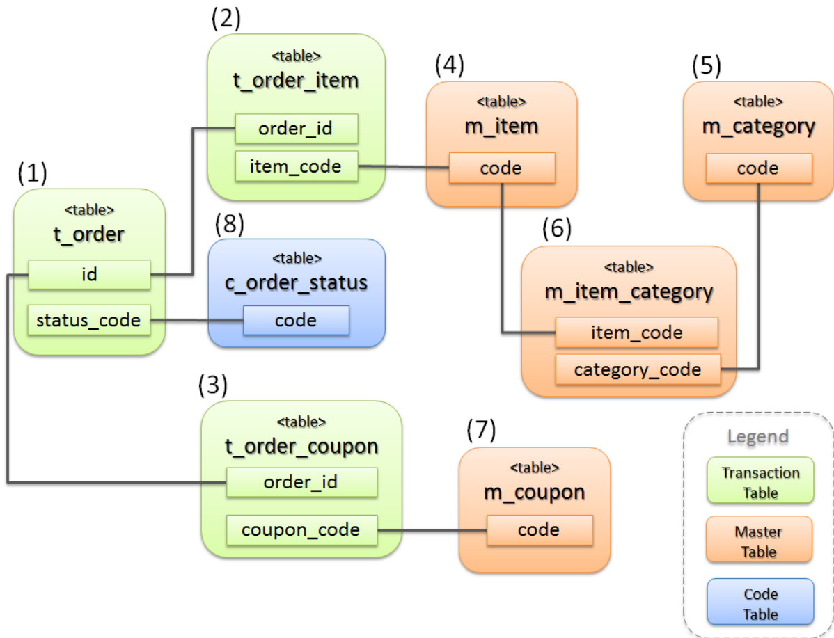
図 6.6 Picture - ER diagram
