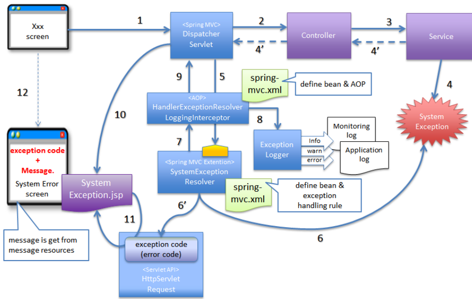
図 4.11 図-サーブレット単位でフレームワークがハンドリングする場合の基本フロー
