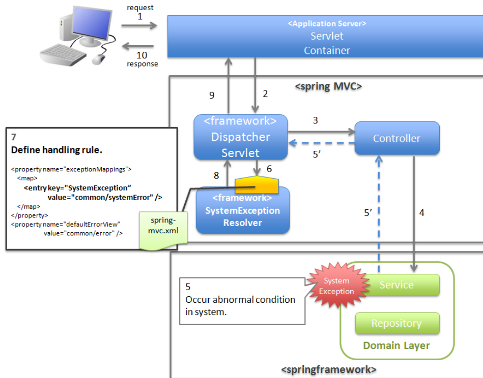
図 4.5 図-システム、またはアプリケーションが、正常な状態でないことを通知する例外を検知する場合のハンドリング方法
