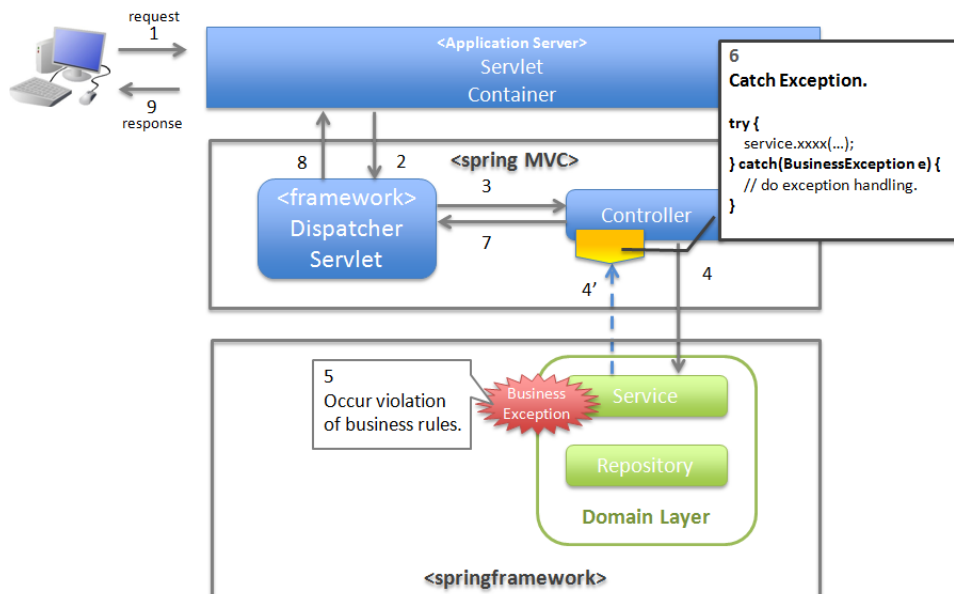
図 4.3 図-ユースケースの一部やり直し (途中からのやり直し) を促す場合のハンドリング方法
