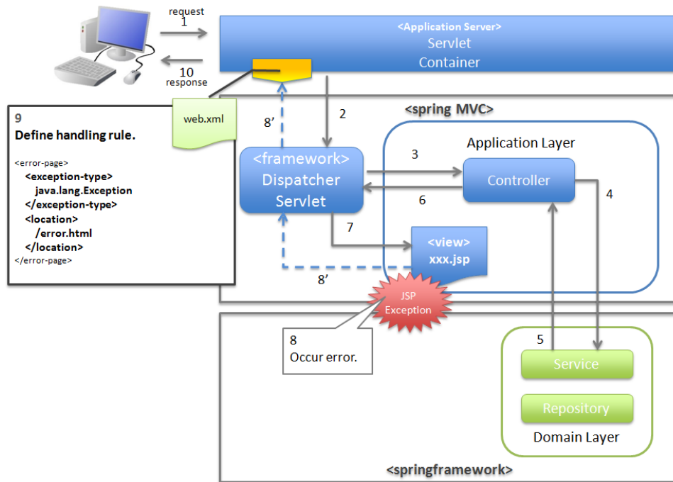
図 4.8 図-プレゼンテーション層 (JSP など) で例外が発生した事を通知する場合のハンドリング方法
