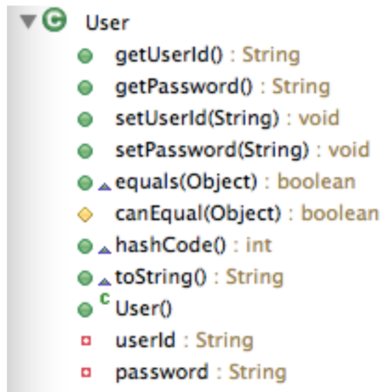
図 11.1 Lombok によって生成されたクラス構造
