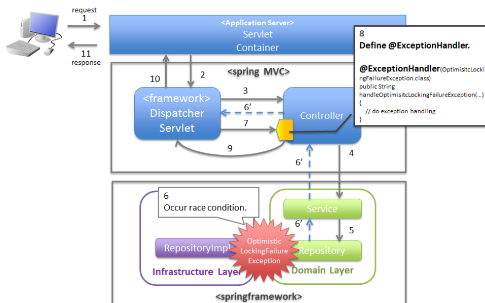
図 4.4 図-ユースケースのやり直し (先頭からのやり直し) を促す場合のハンドリング方法
