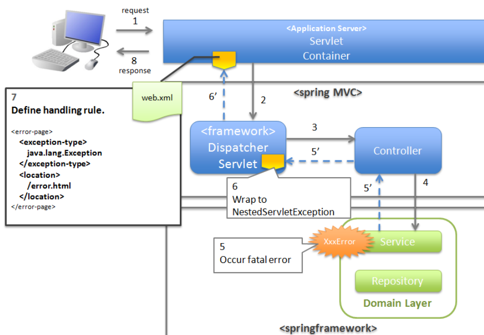
図 4.7 図-致命的なエラーが発生したことを検知する場合のハンドリング方法
