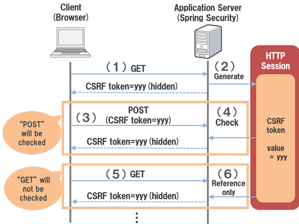
図 9.9 Spring Security の CSRF 対策の仕組み
