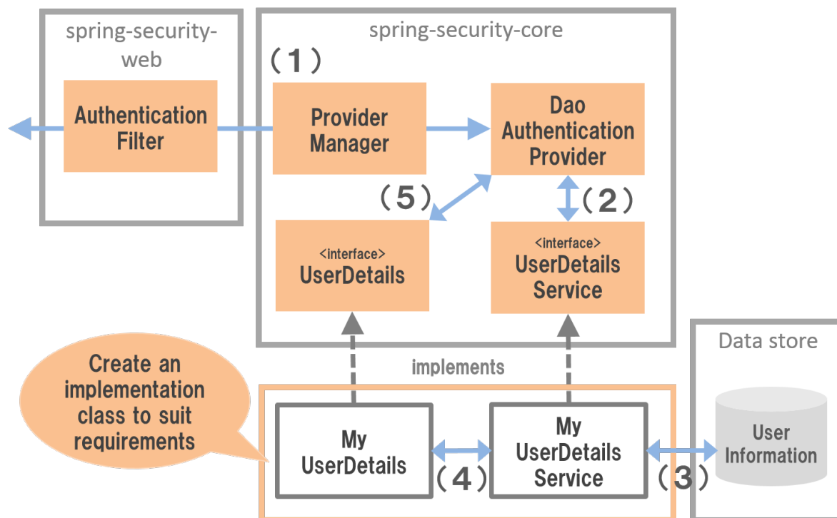
図 9.4 DB 認証の仕組み
