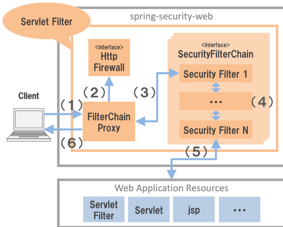
図 9.1 Spring Security のフレームワークアーキテクチャ
