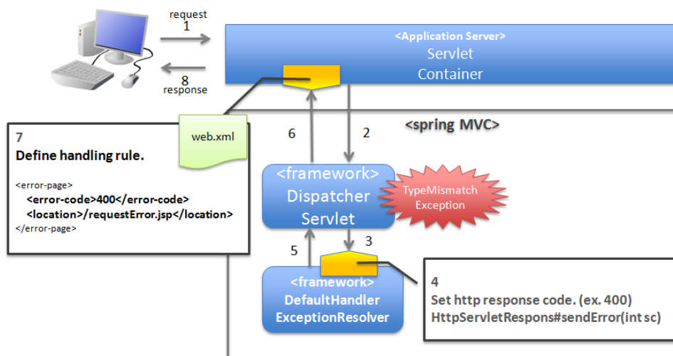
図 4.6 図-リクエスト内容が不正であることを通知する場合のハンドリング方法
