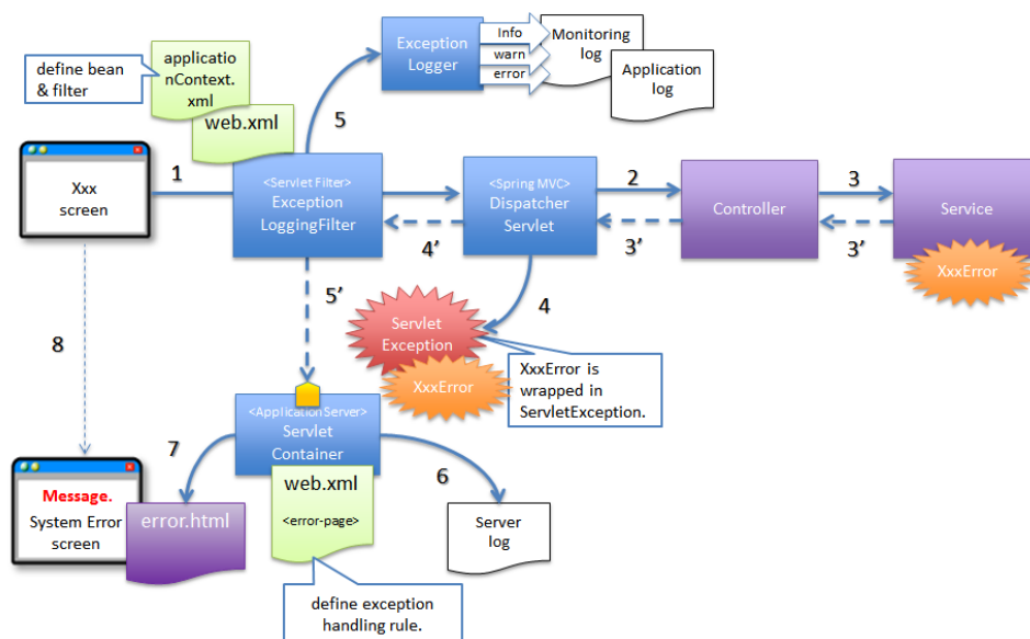
図 4.12 図-Web アプリケーション単位でサーブレットコンテナがハンドリングする場合の基本フロー
