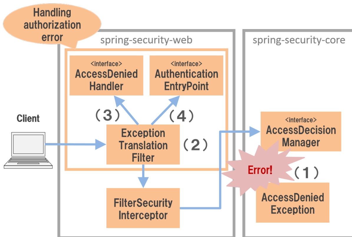
図 9.8 認可エラーのハンドリングの仕組み
