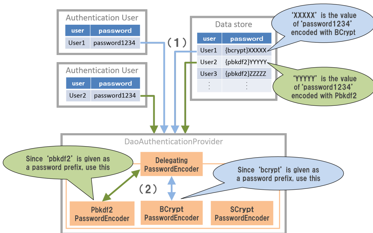
図 5 DelegatingPasswordEncoder の解説
